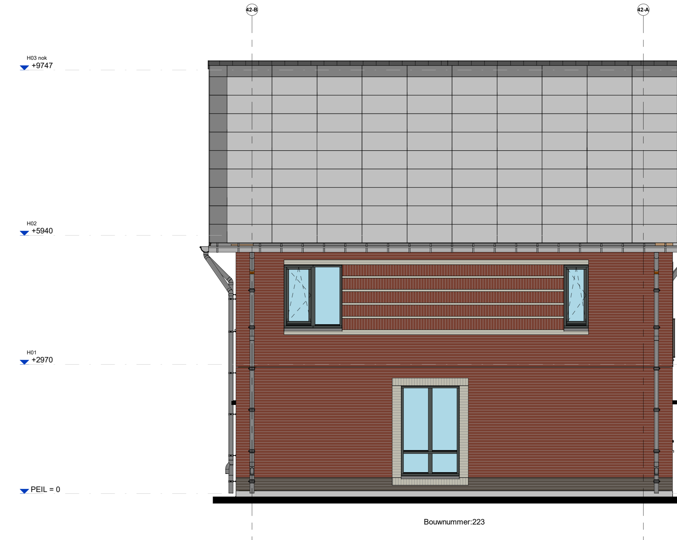
Blok 42 - Linkergevel
