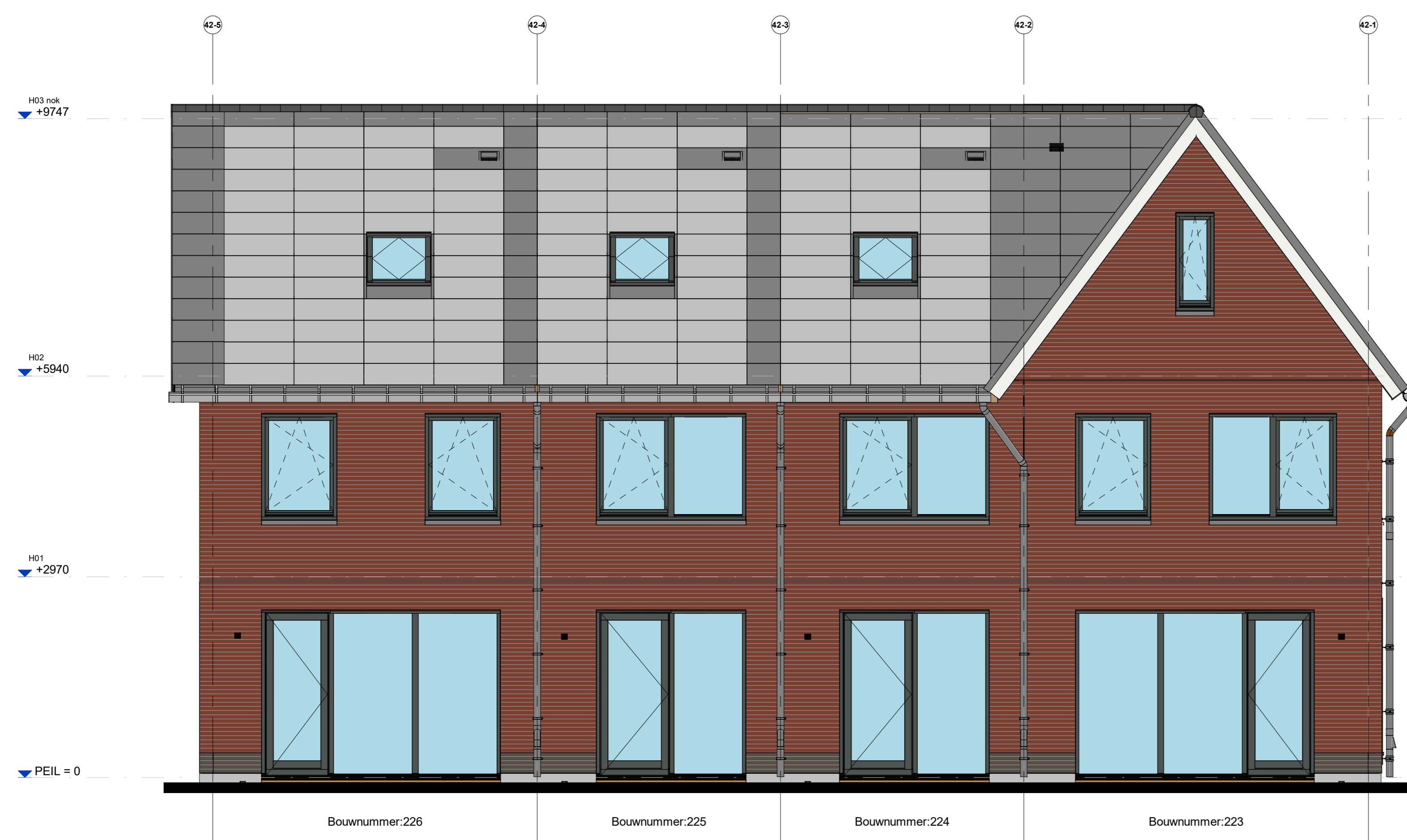
Blok 42 - Achtergevel
