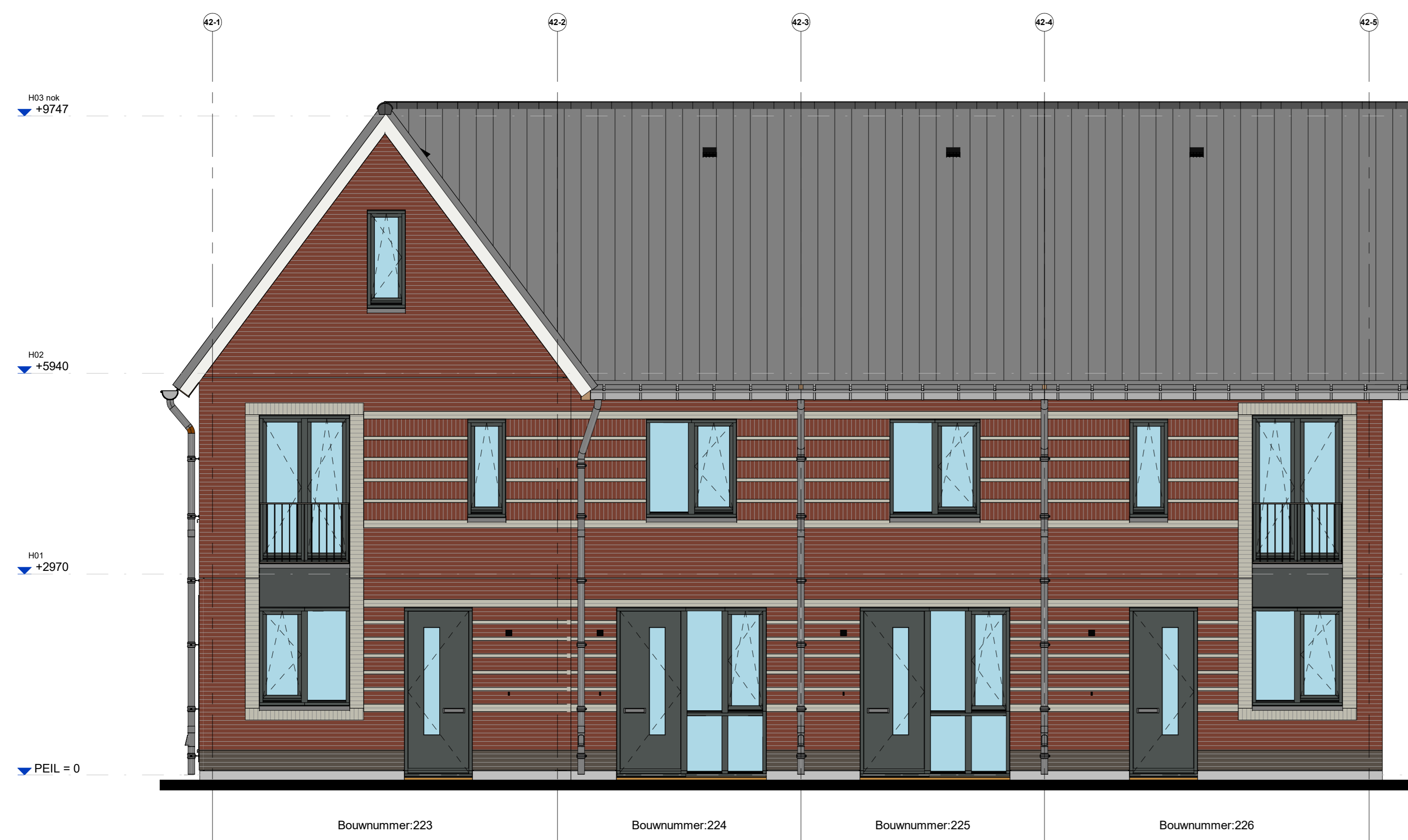
Blok 42 - Voorgevel
