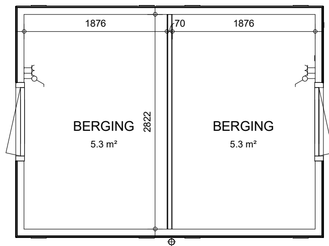
Plattegrond
