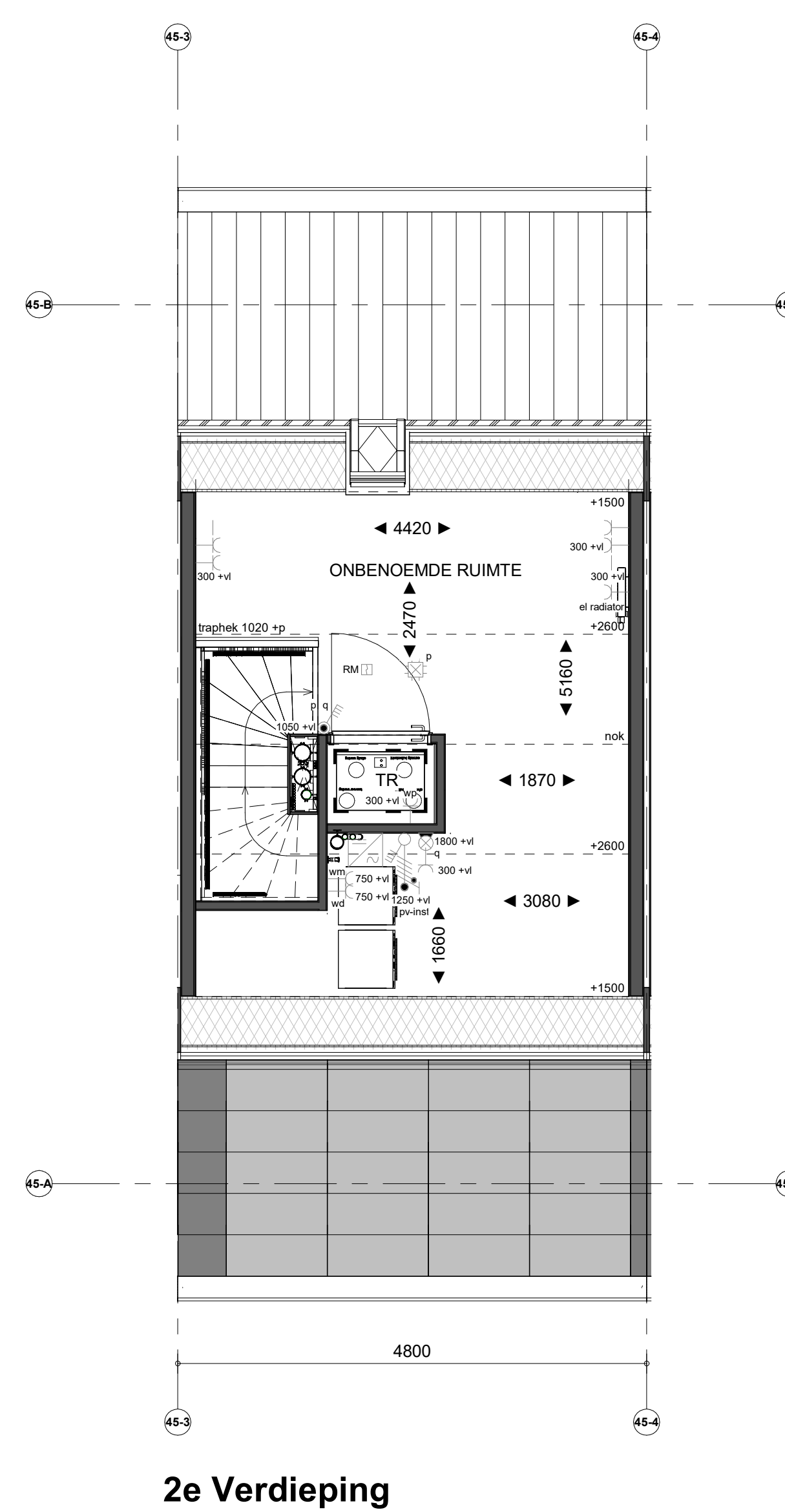
2e Verdieping
