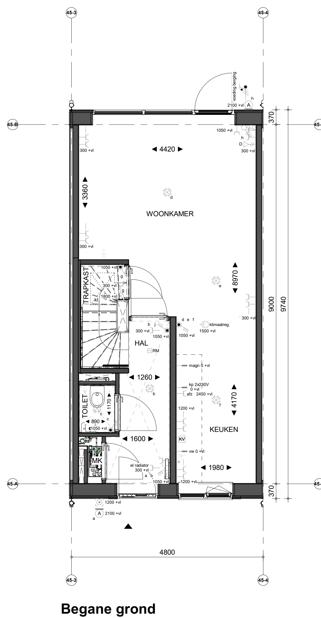
Begane grond
