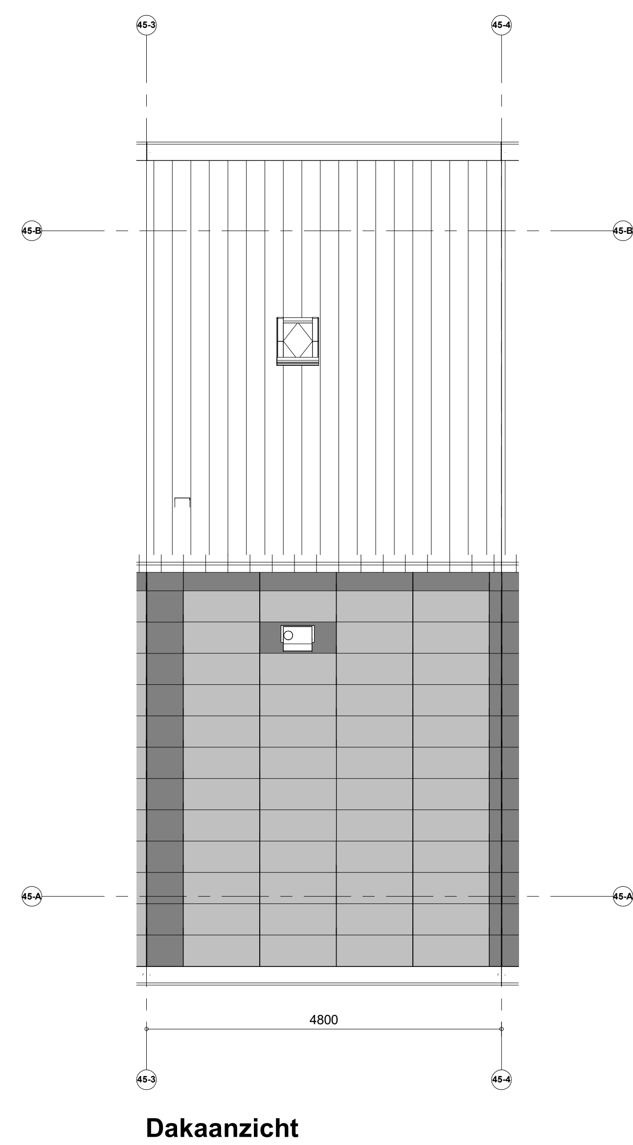
Dakaanzicht
