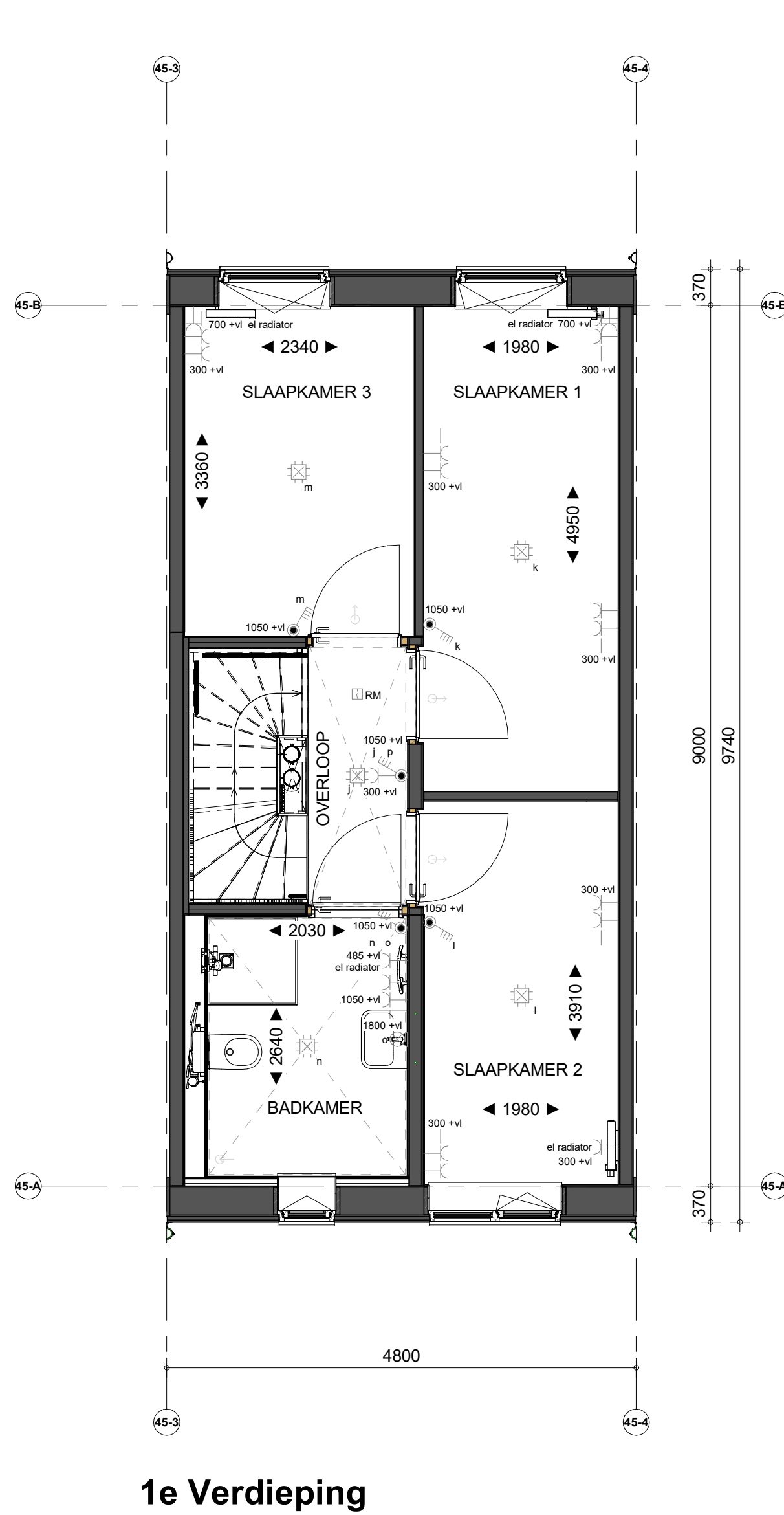
1e Verdieping
