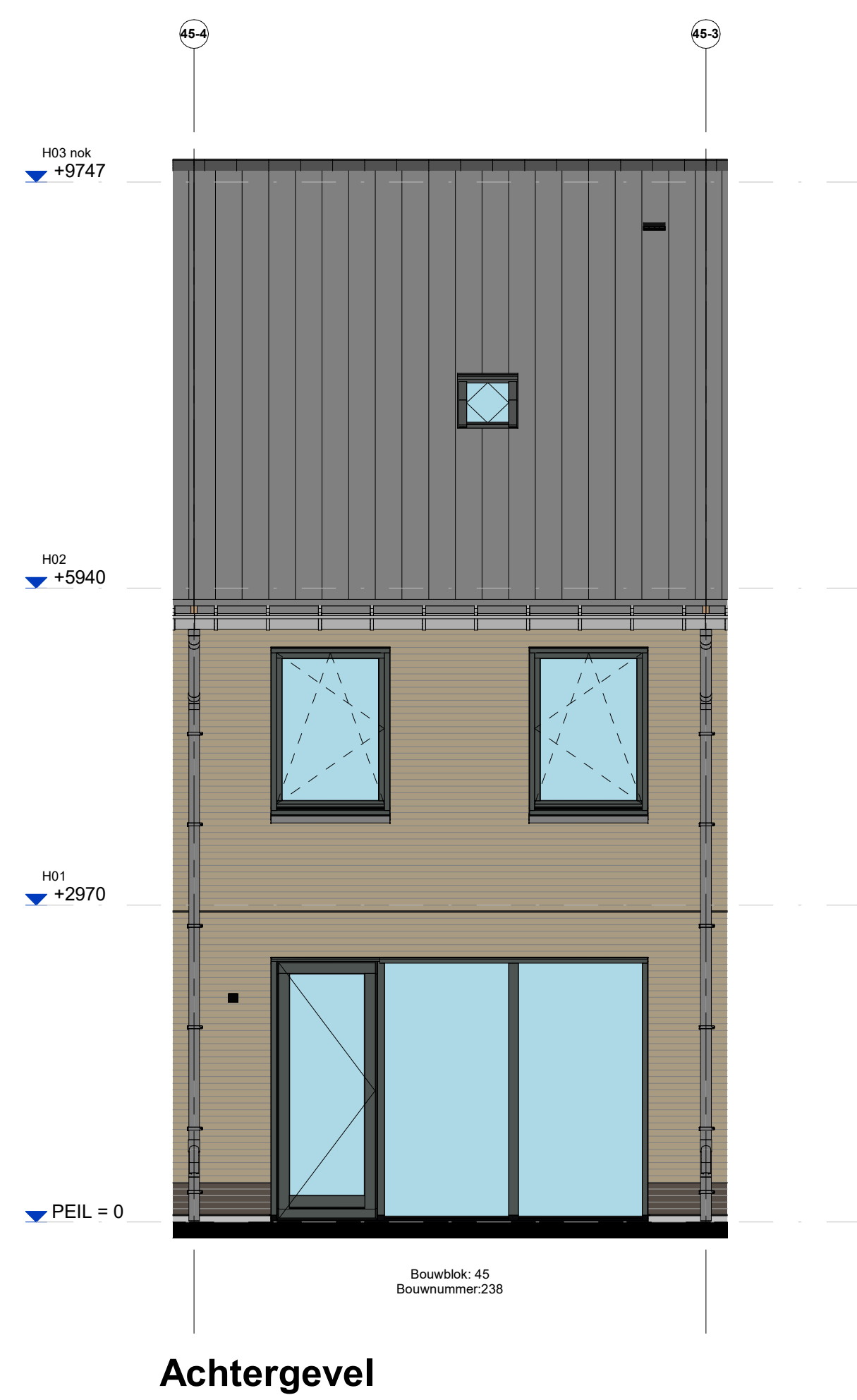
Achtergevel
