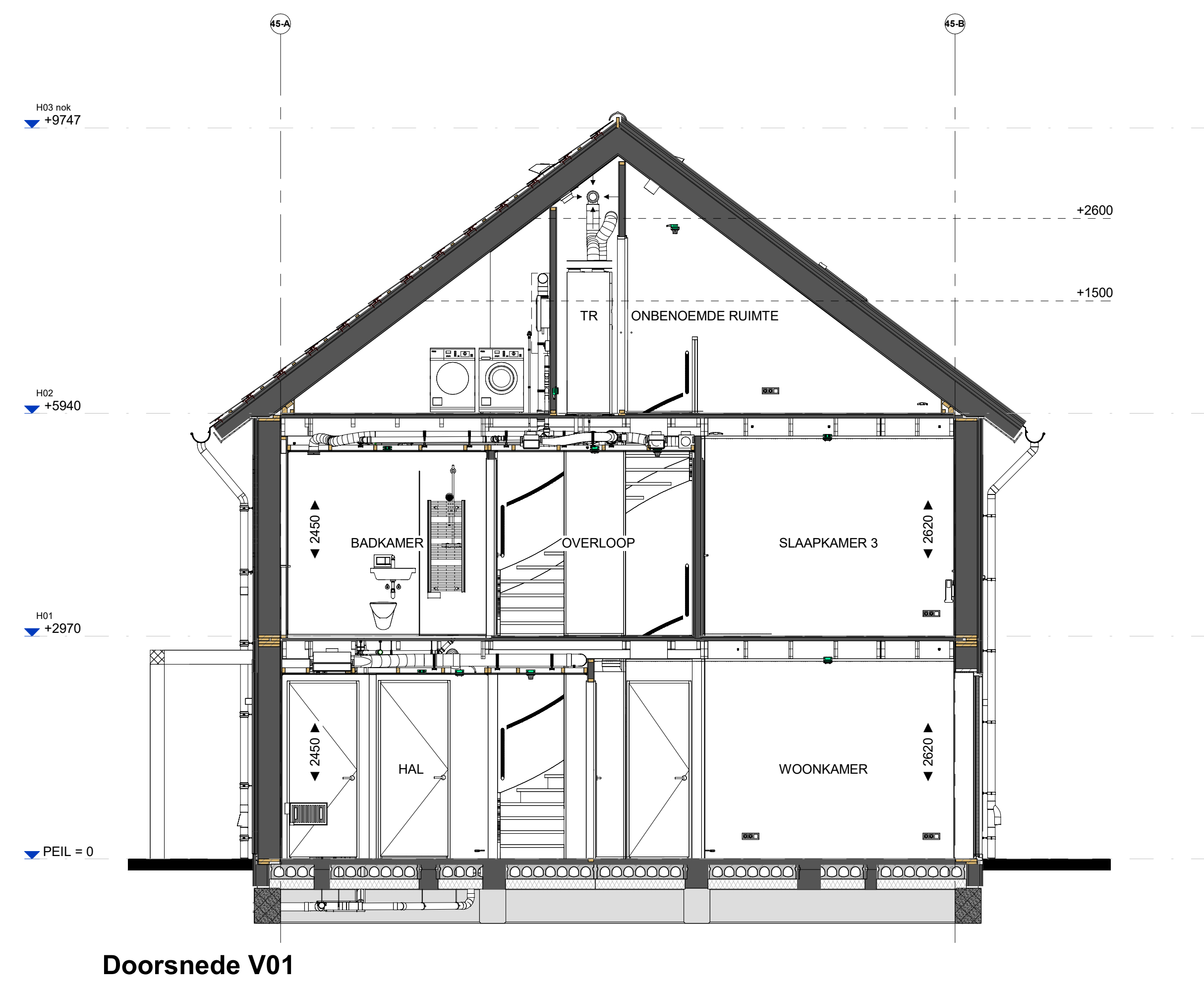
Doorsnede V01
