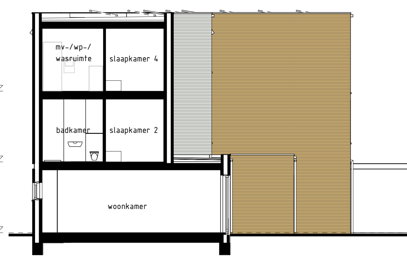
type E1sp bwnr get.:532, 632 DOORSNEDE 9C-9C
