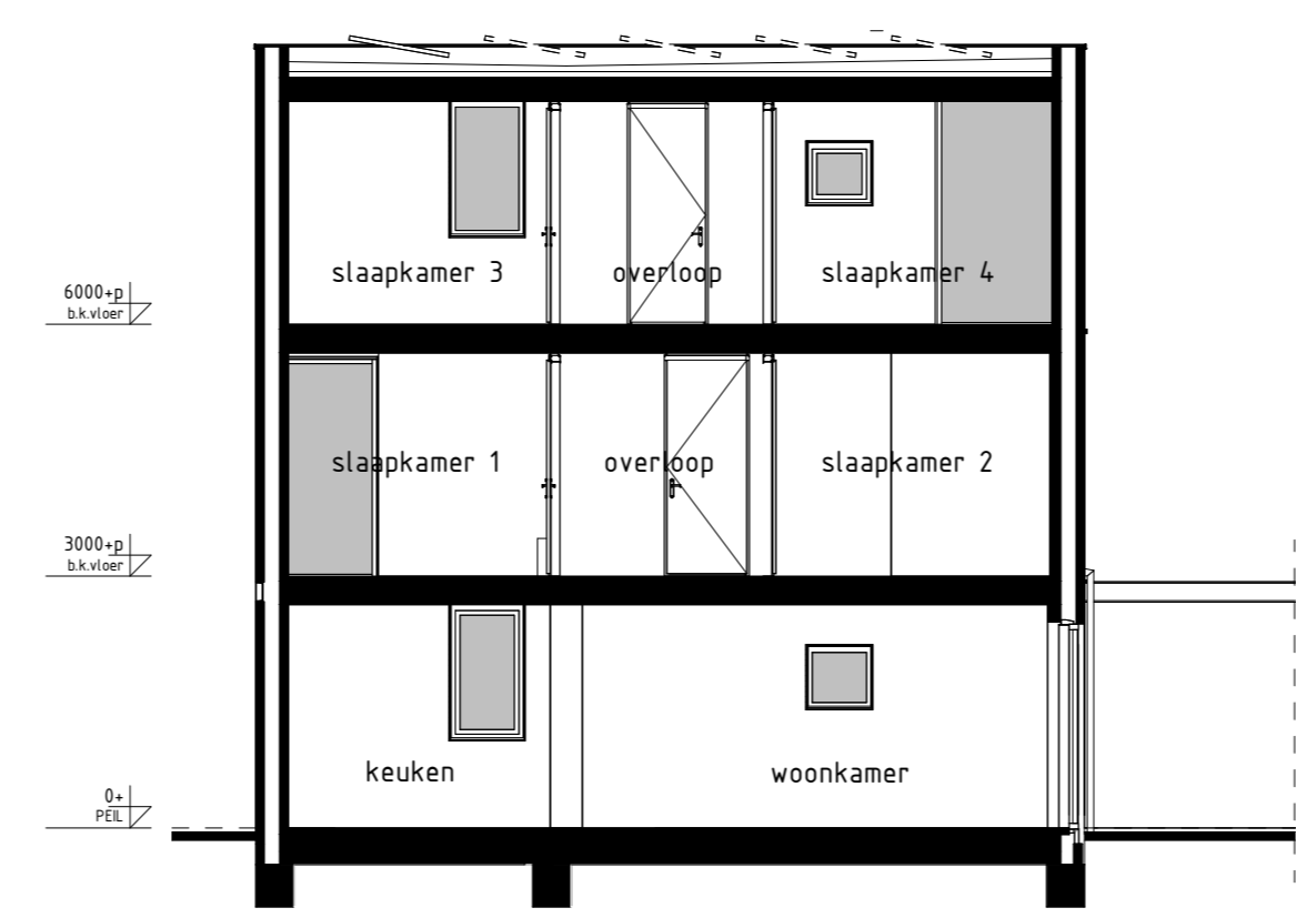
type G1sp bwnr get.:527, 627 DOORSNEDE 9E-9E
