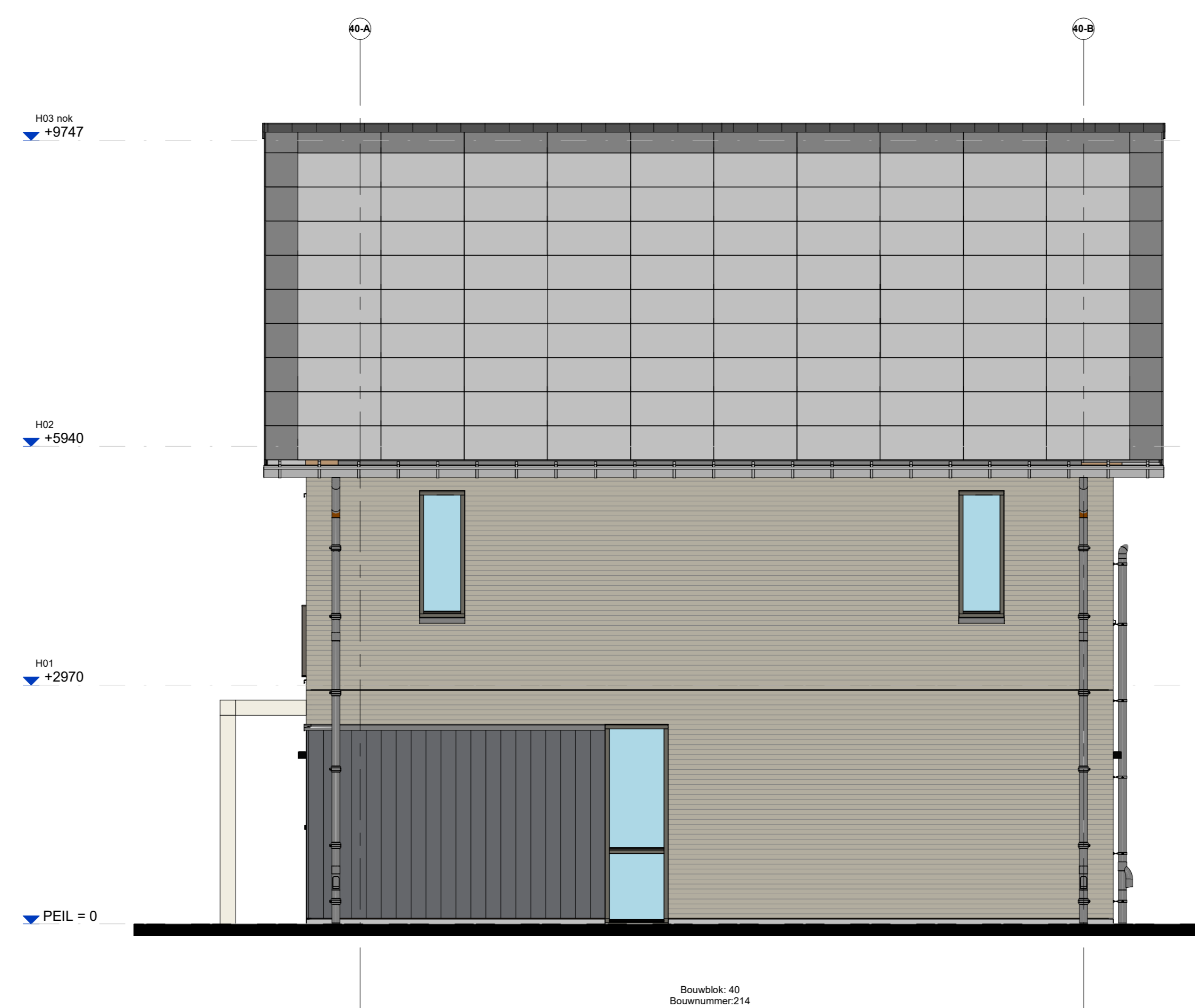
Rechterzijgevel
