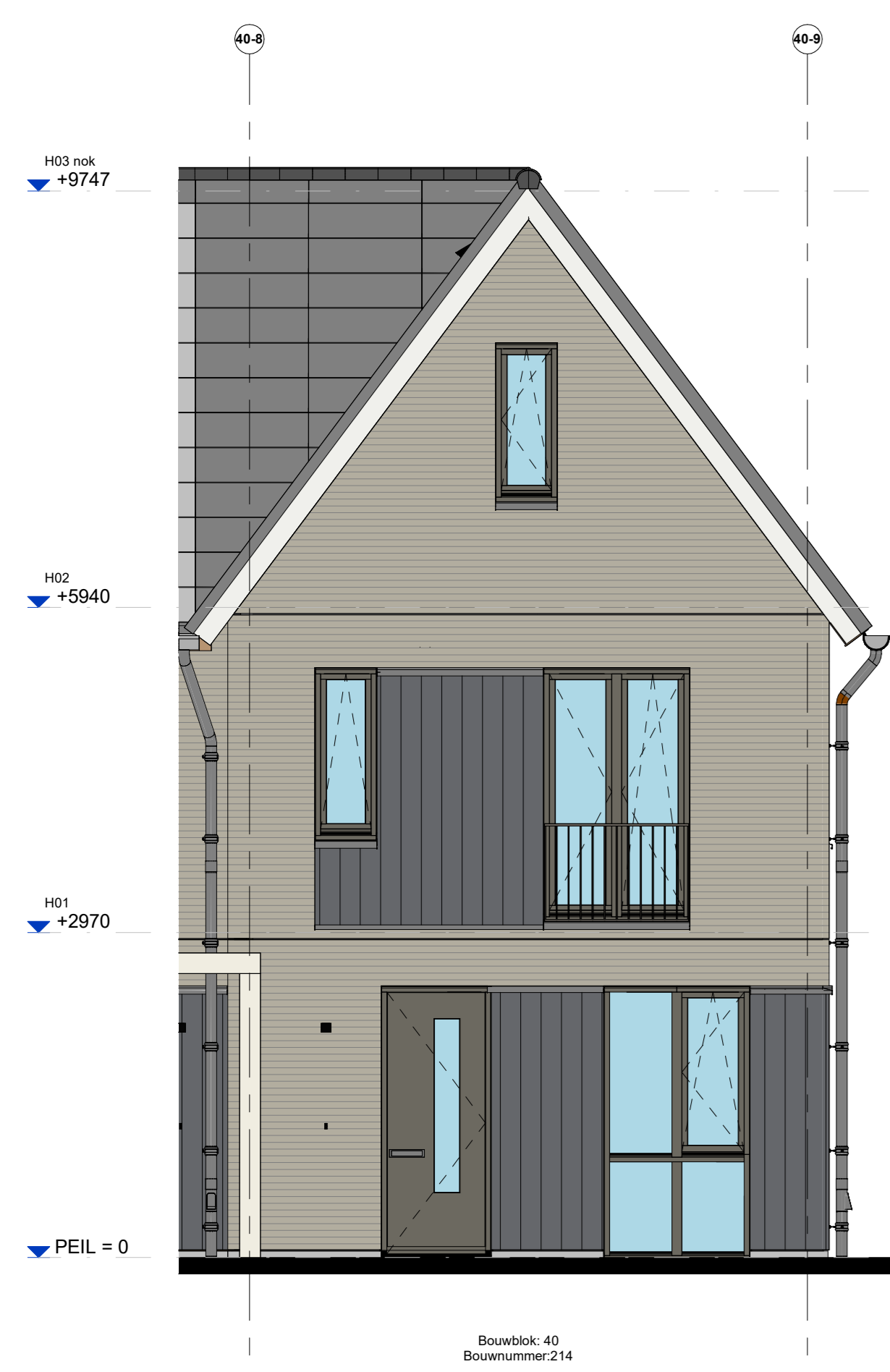
Voorgevel
