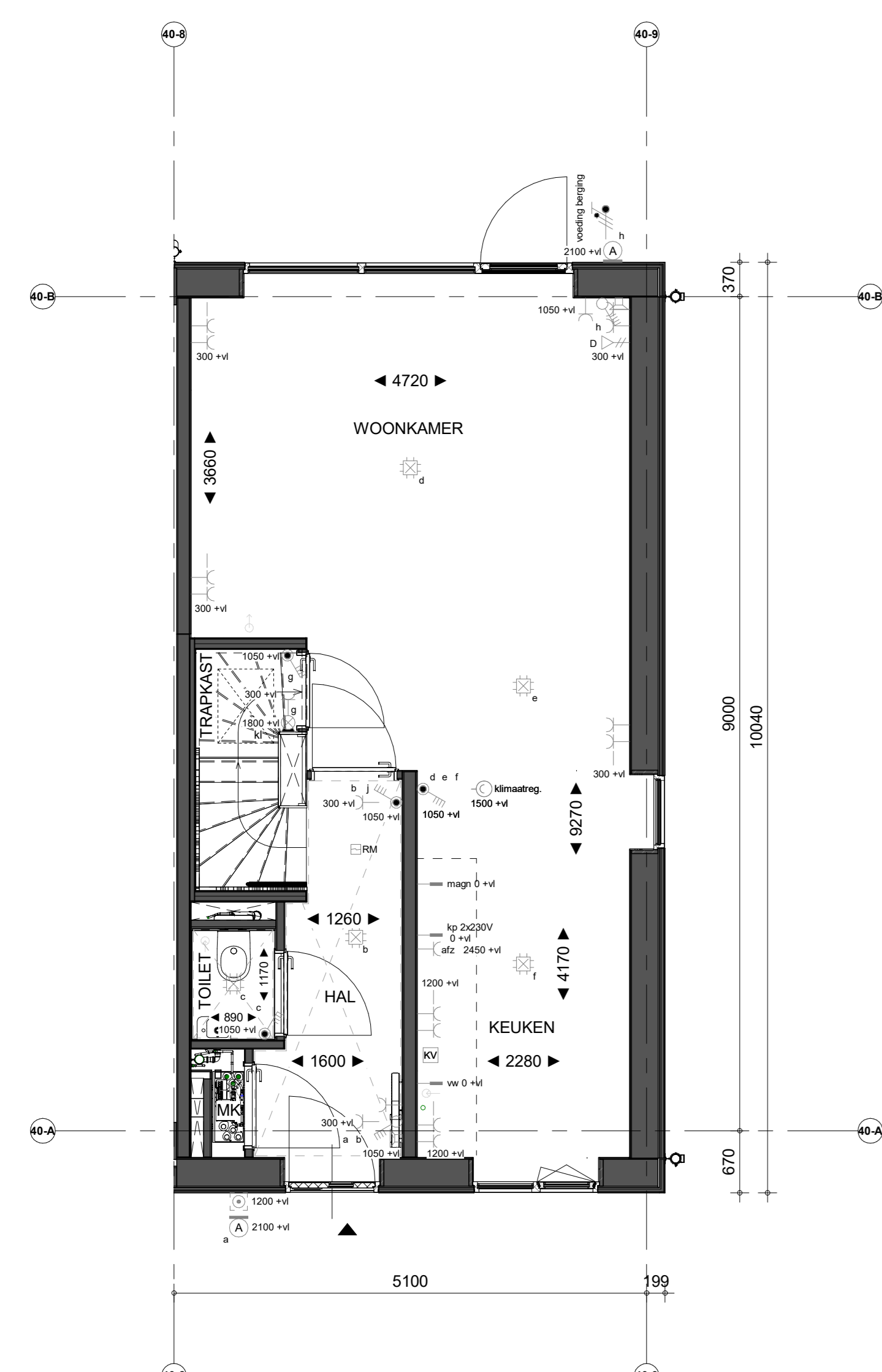
Begane grond
