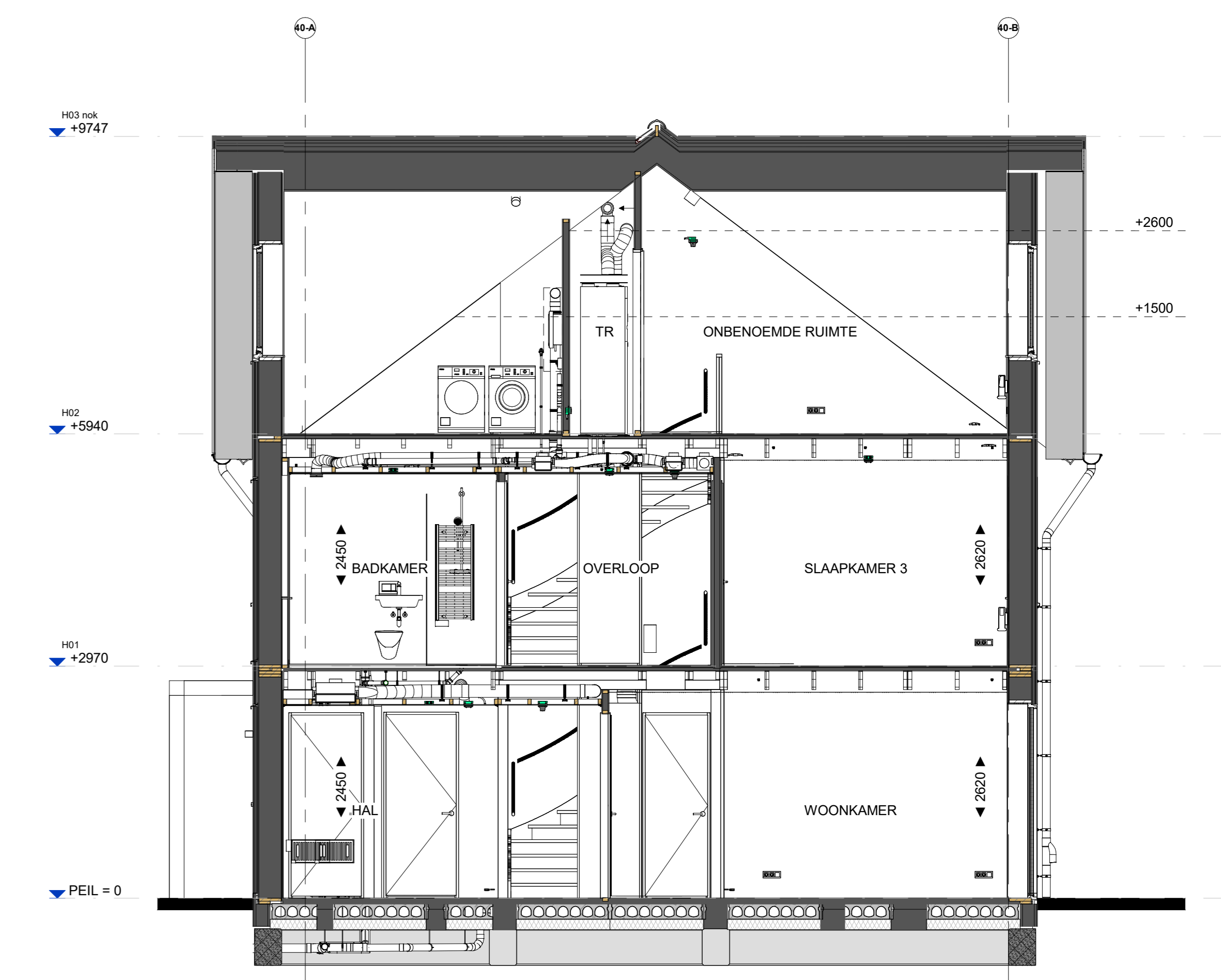
Doorsnede V01
