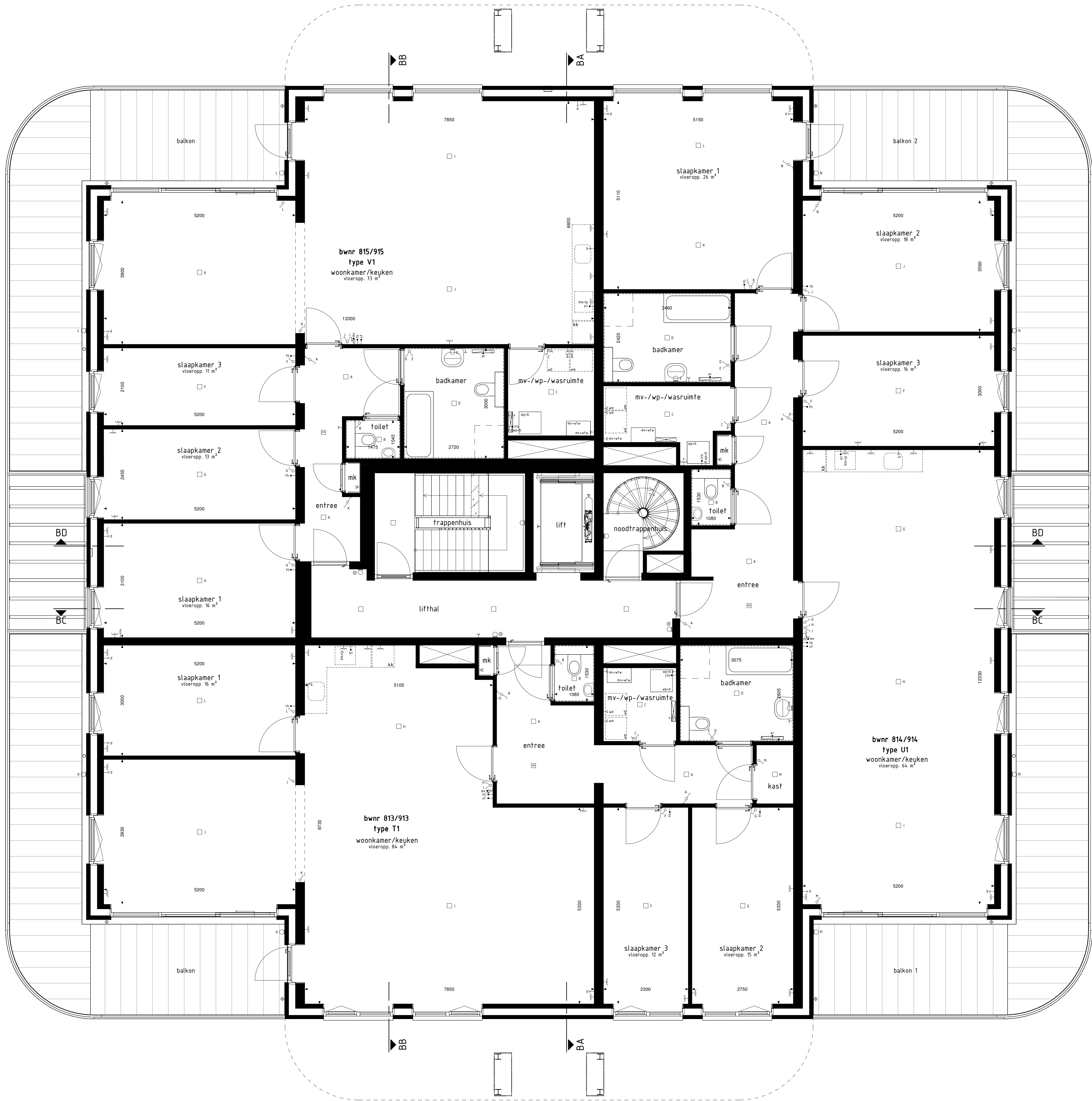
3e VERDIEPING
