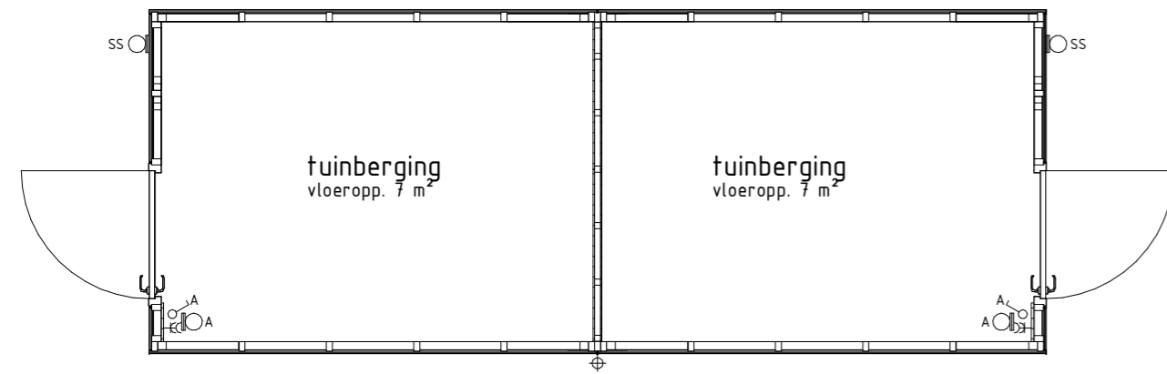
PLATTEGROND
