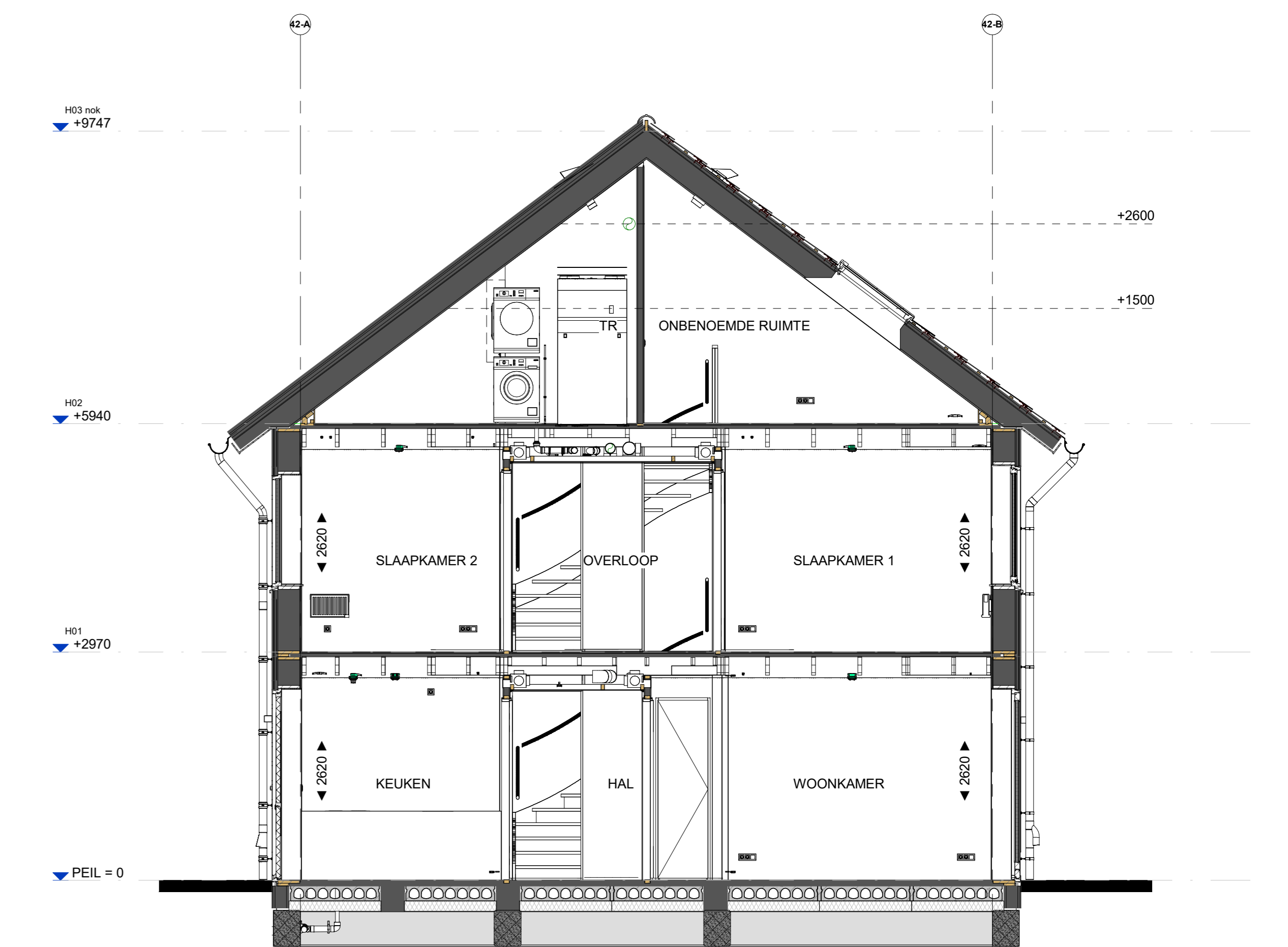
Doorsnede V01
