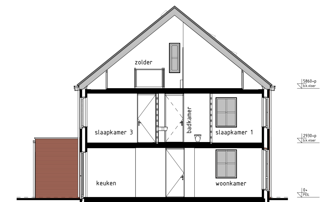
type M1sp bwnr get.:54 DOORSNEDE M1sp-M1sp
