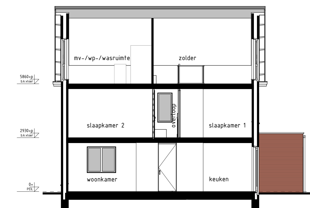
type W1 bwnr get.:53 DOORSNEDE W1-W1
