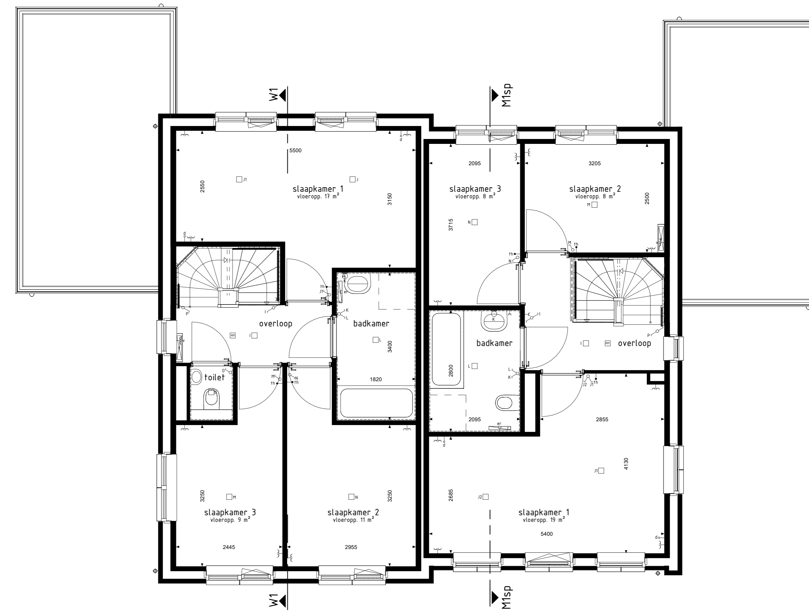
type W1 bwnr get.:53
