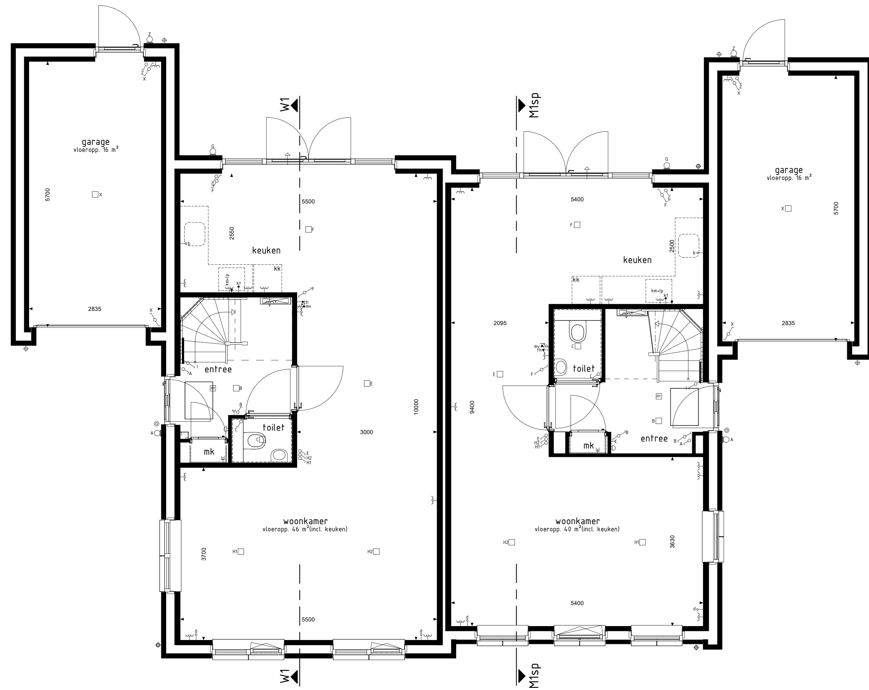
type W1 bwnr get.:53
