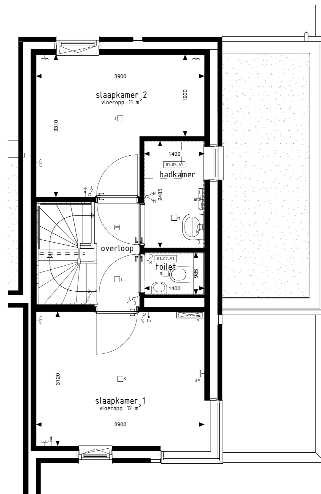
1e VERDIEPING 1:50
