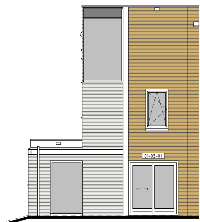
ACHTERGEVEL 1:100
