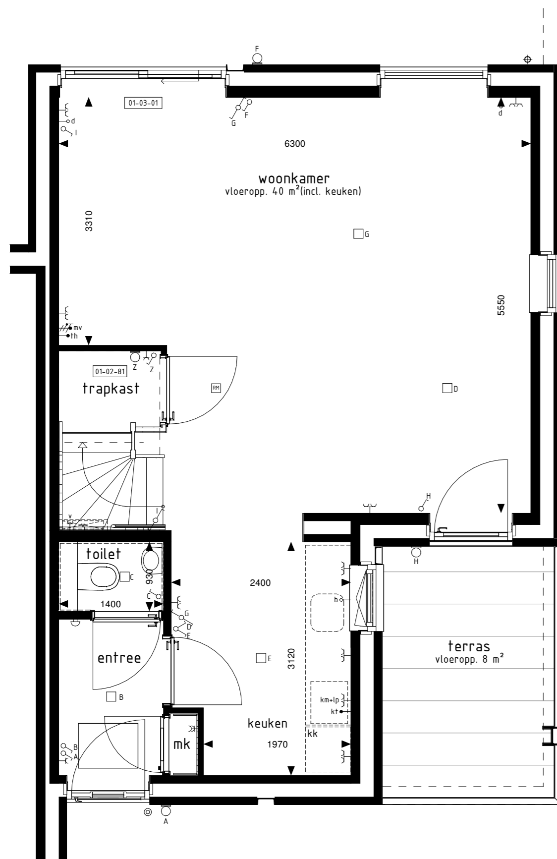
BEGANE GROND 1:50
