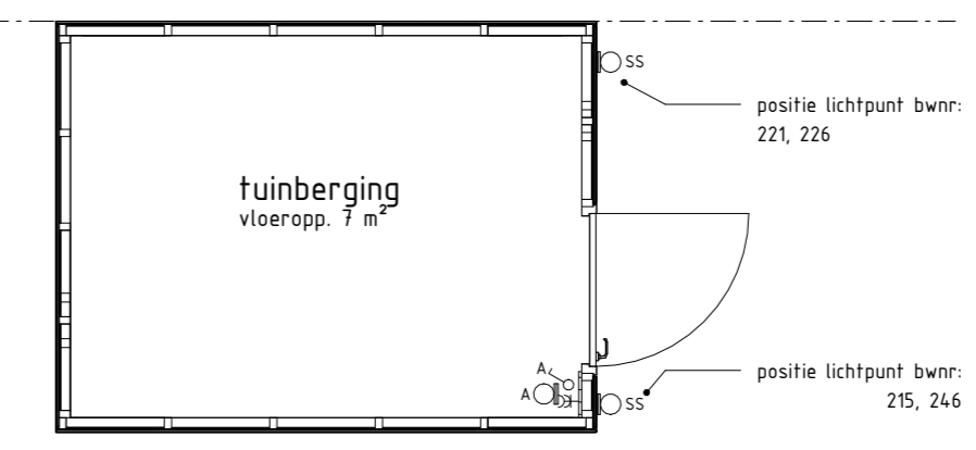
PLATTEGROND bwnr get.: 221 bwnr gesp.: 215, 226, 246
