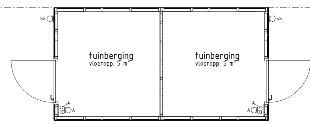
PLATTEGROND bwnr get.: 238, 240 bwnr get.: 239, 241
