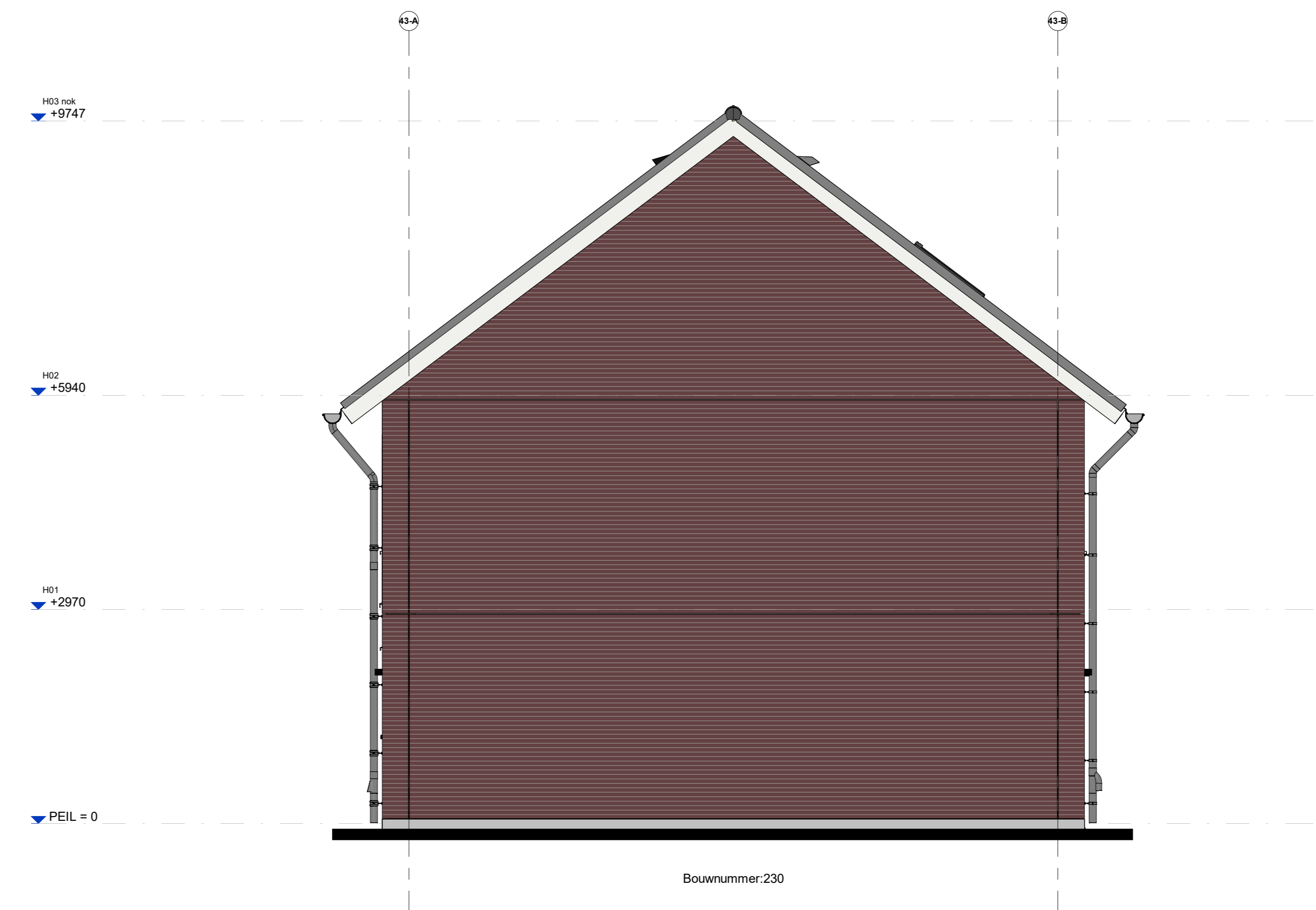
Blok 43 - Rechtergevel
