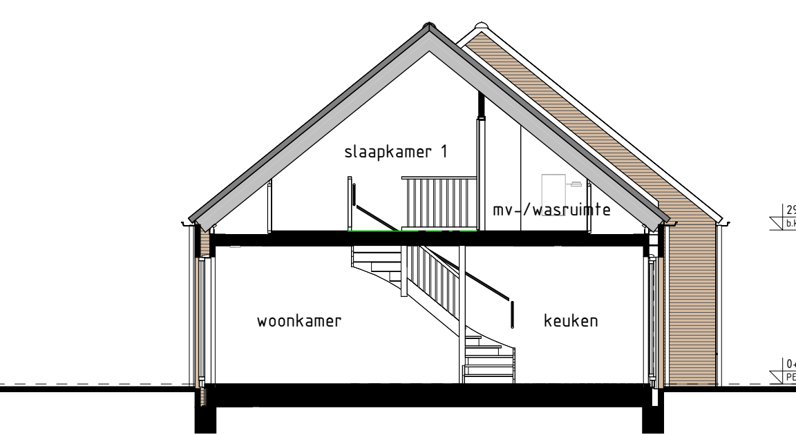
type A2, A2sp, A3sp bwnr get.:132 bwnr gesp.:131, 133 DOORSNEDE A2-A2 1:100
