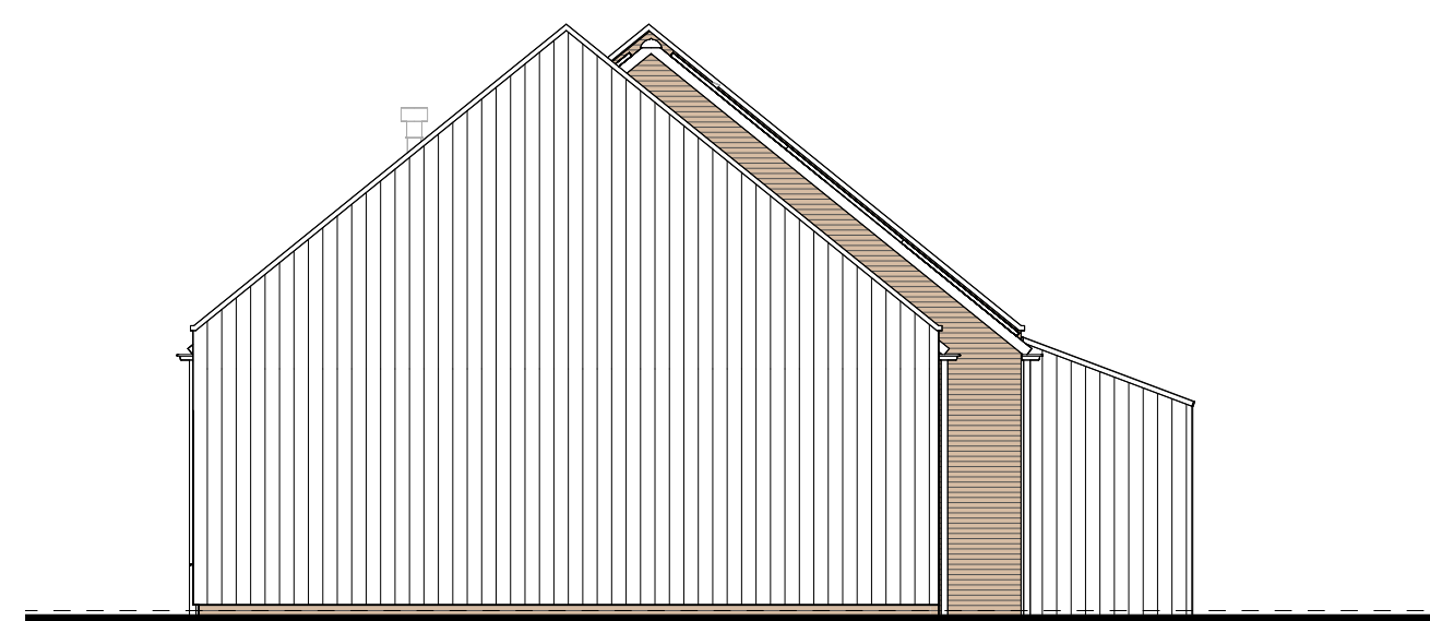
type B3 bwnr get.:134 RECHTERGEVEL 1:100
