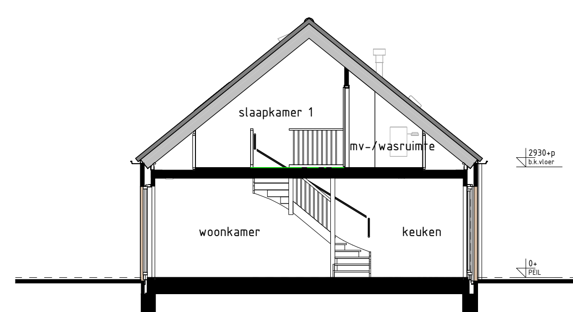
type B2, B3 bwnr get.:130, 134 DOORSNEDE B2-B2 1:100
