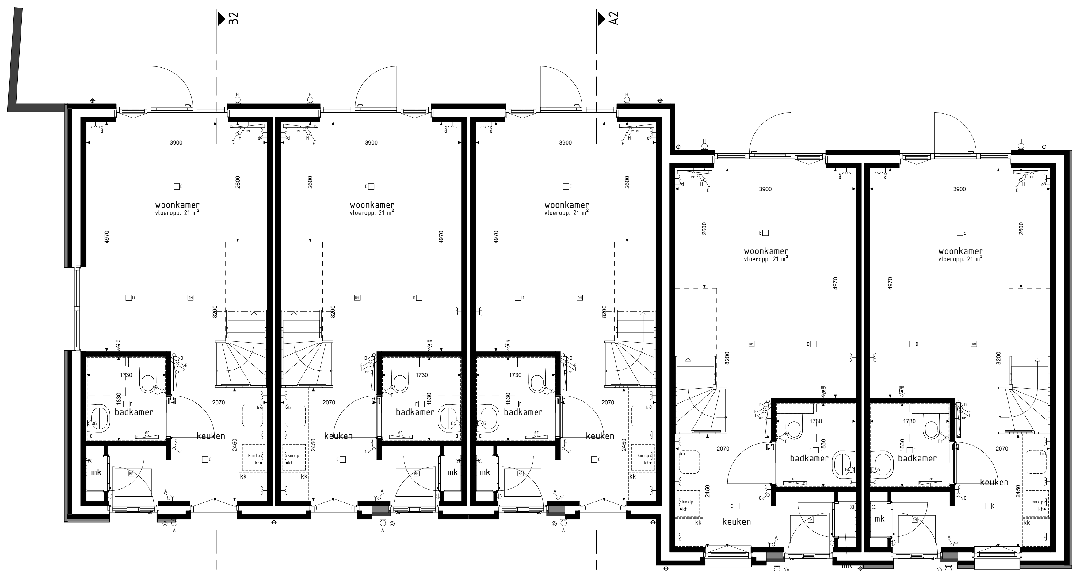
type B2 bwnr get.:130 type A2sp bwnr get.:131 type A2 bwnr get.:132 type A3sp bwnr get.:133 type B3 bwnr get.:134 BEGANE GROND 1:50
