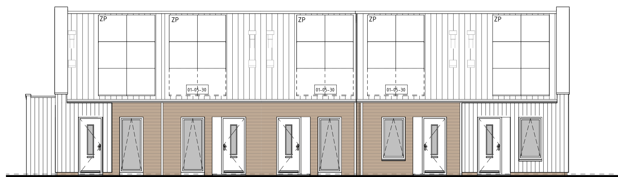
type B2 bwnr get.:130 type A2sp bwnr get.:131 type A2 bwnr get.:132 type A3sp bwnr get.:133 type B3 bwnr get.:134 VOORGEVEL 1:100
