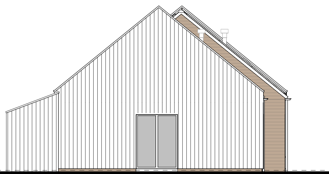
type B2 bwnr get.:130 LINKERGEVEL 1:100
