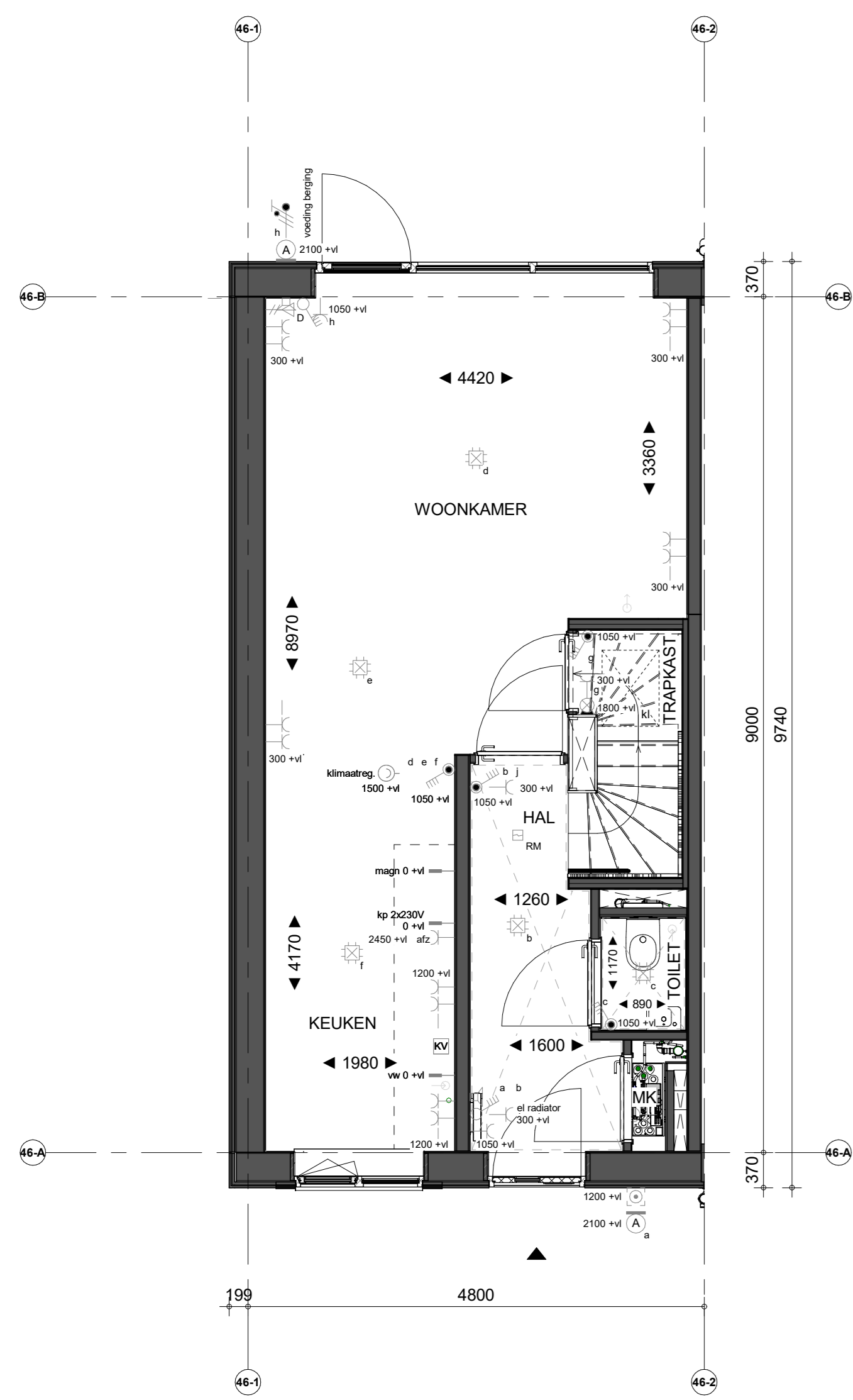
Begane grond
