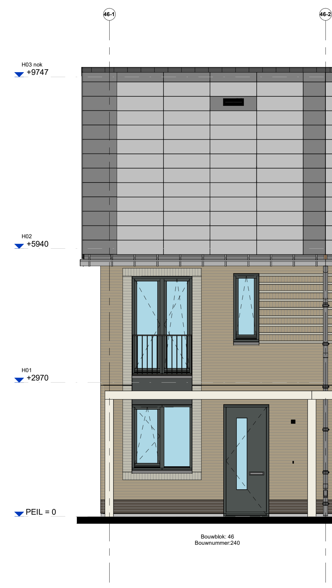
Voorgevel
