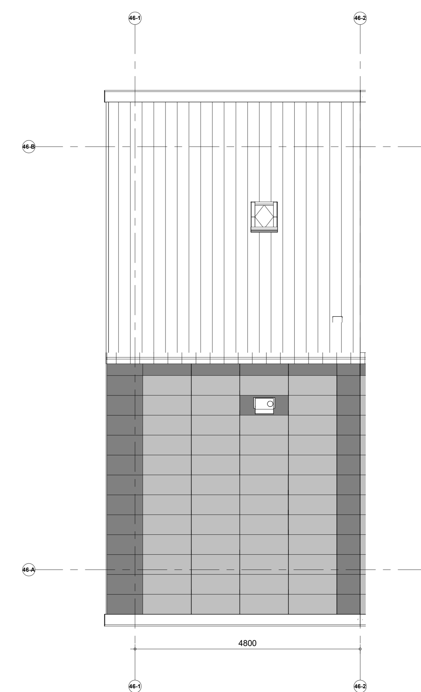
Dakaanzicht
