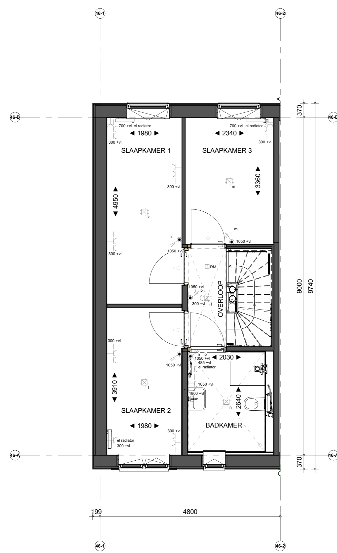
1e Verdieping
