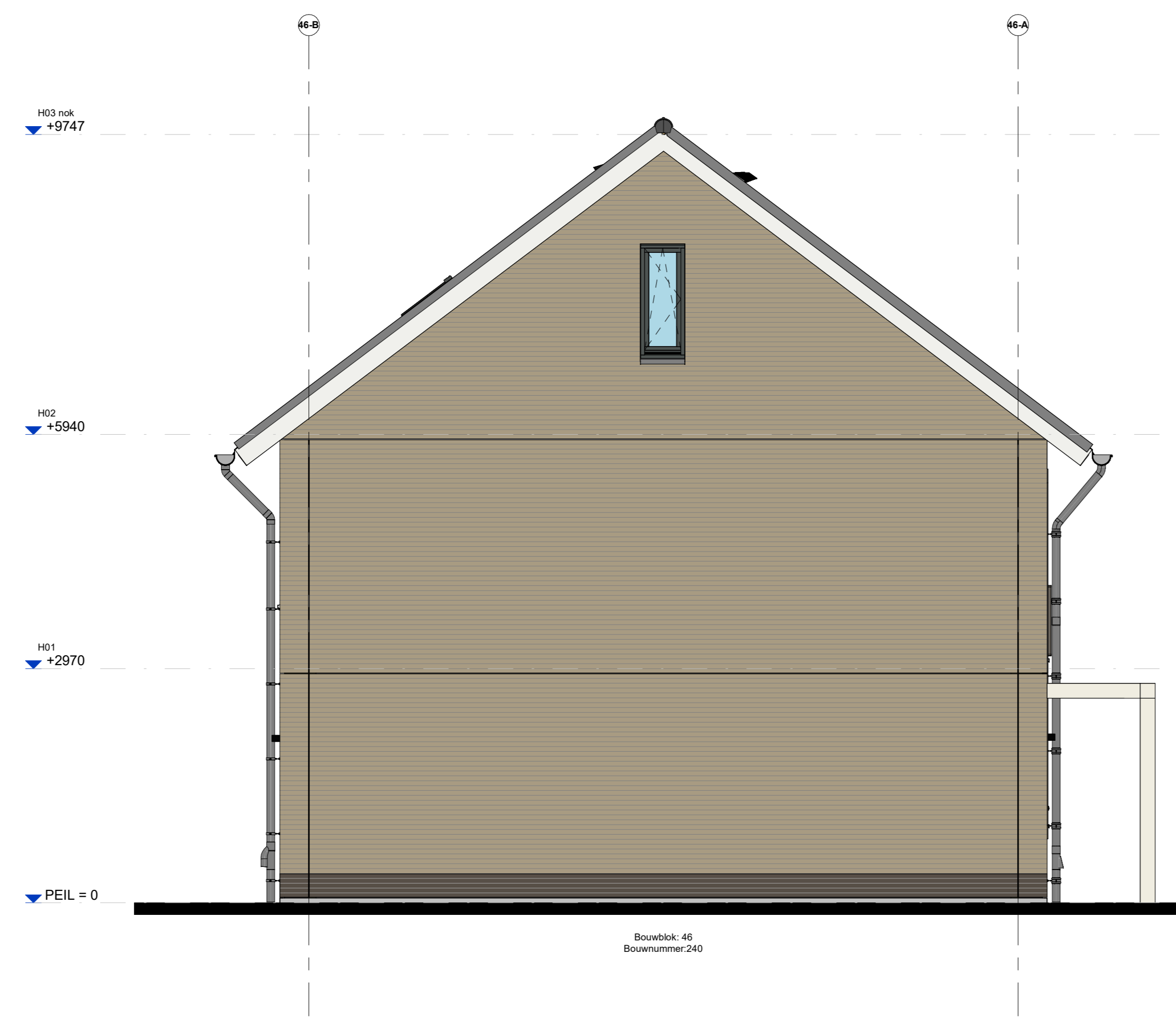
Linkerzijgevel
