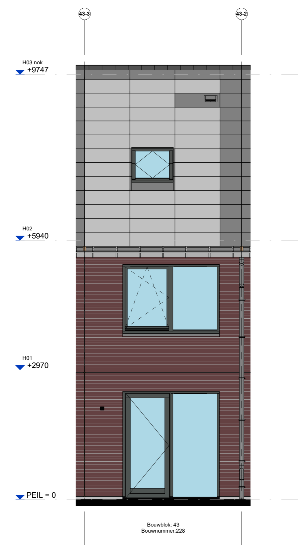
Achtergevel
