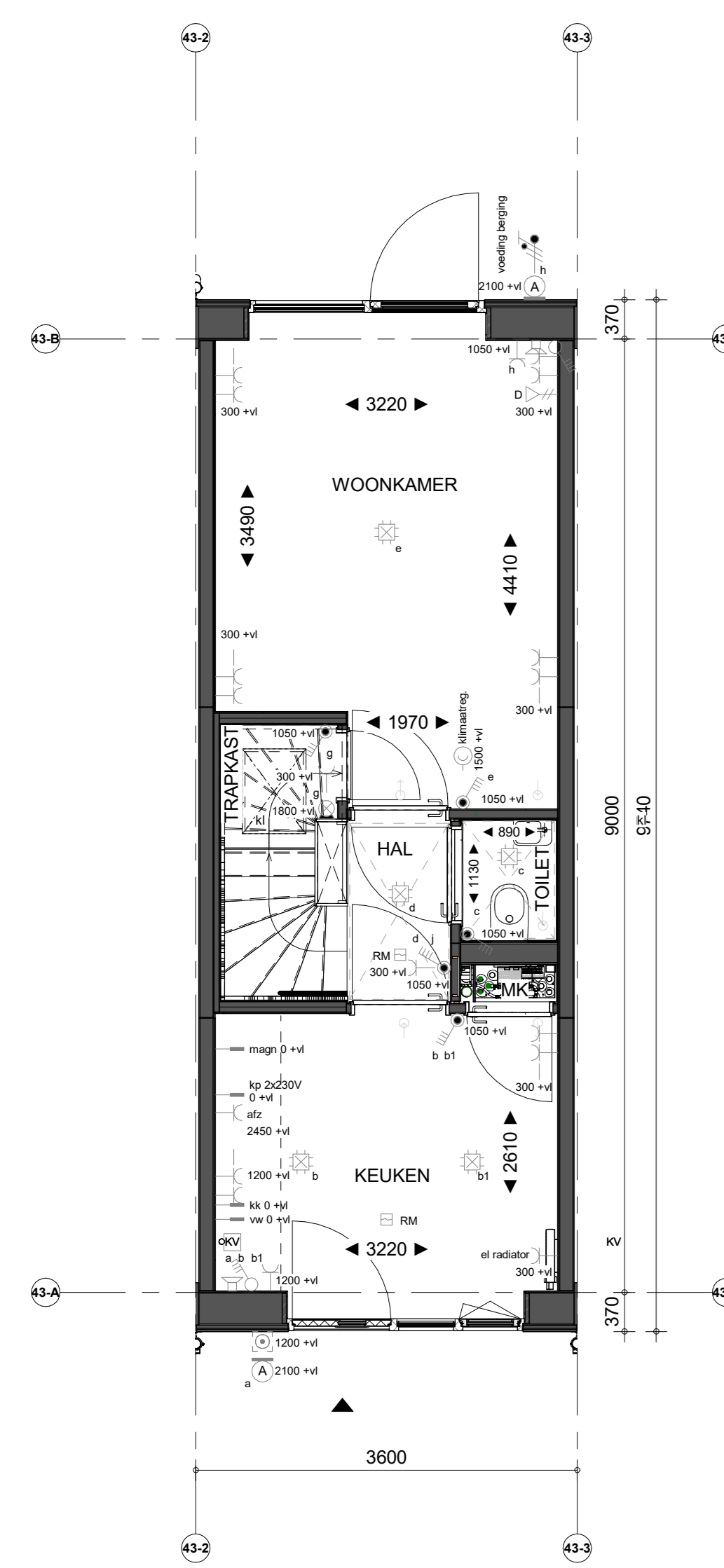
Begane grond
