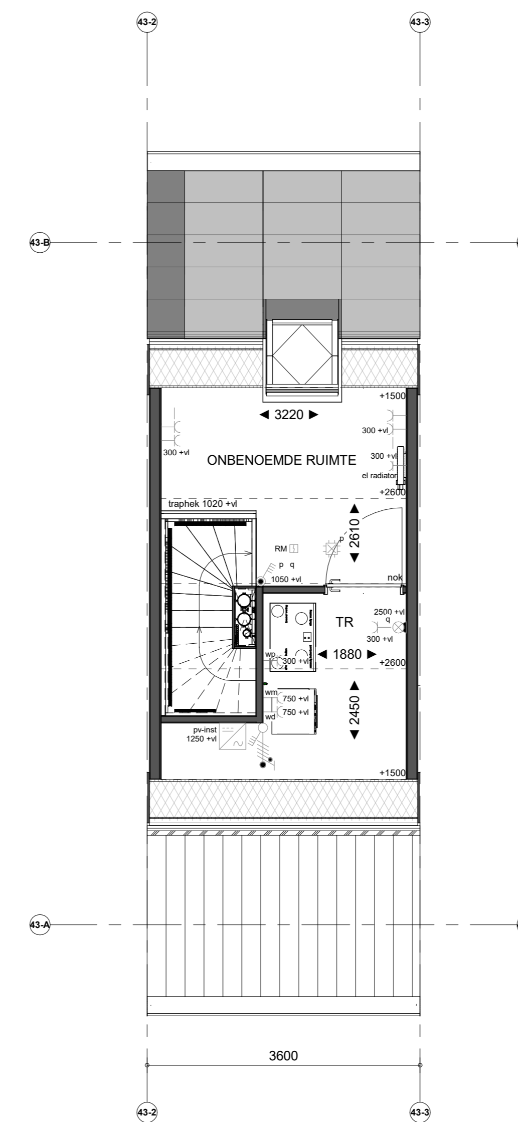
2e Verdieping
