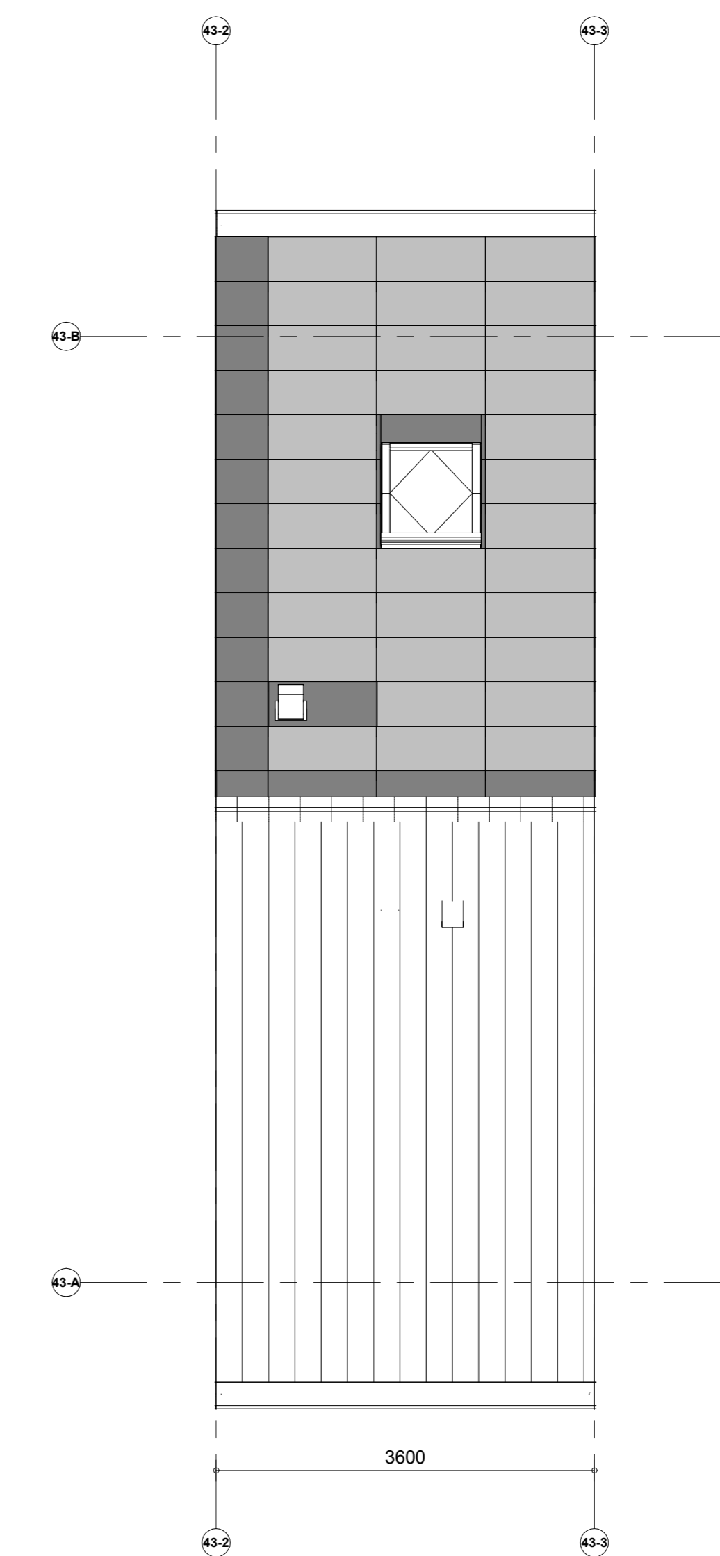
Dakaanzicht
