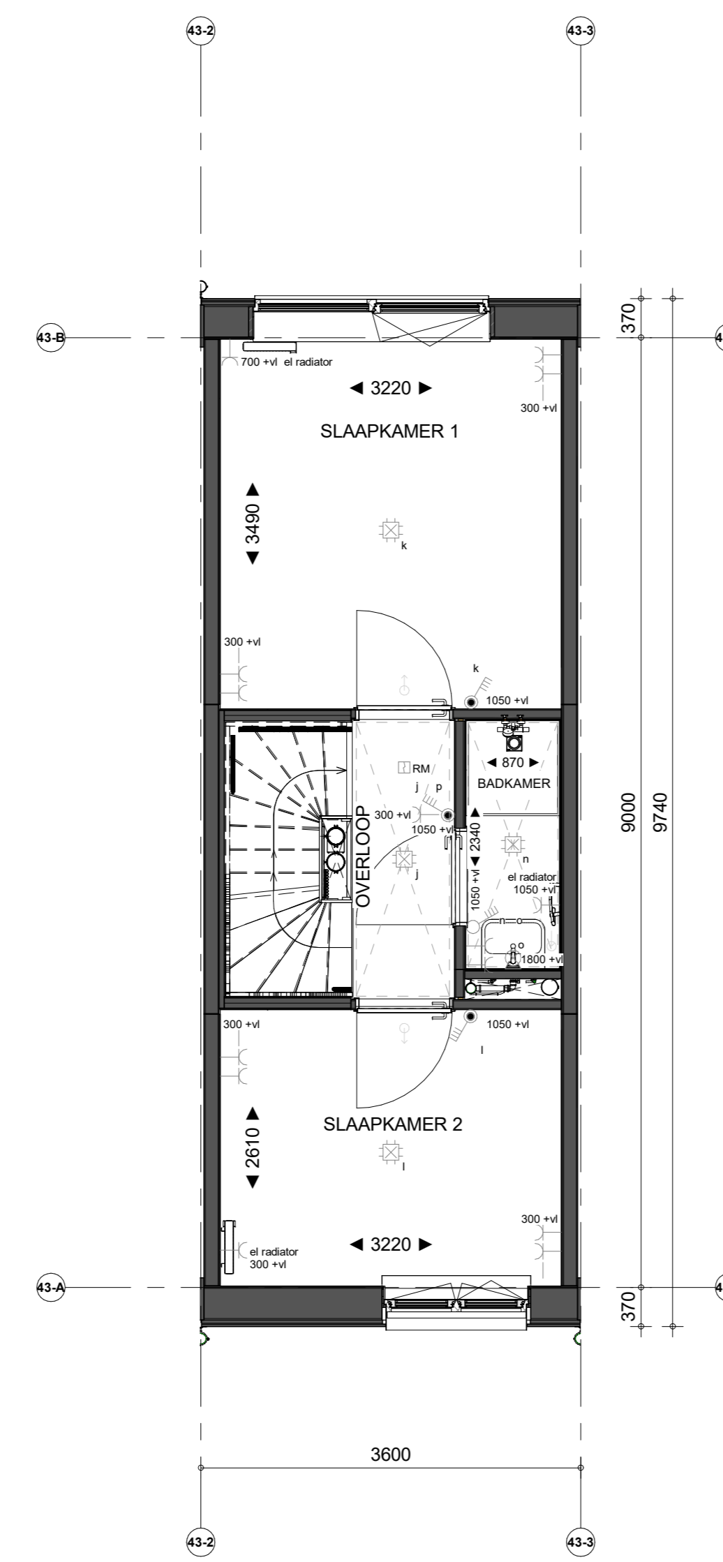
1e Verdieping
