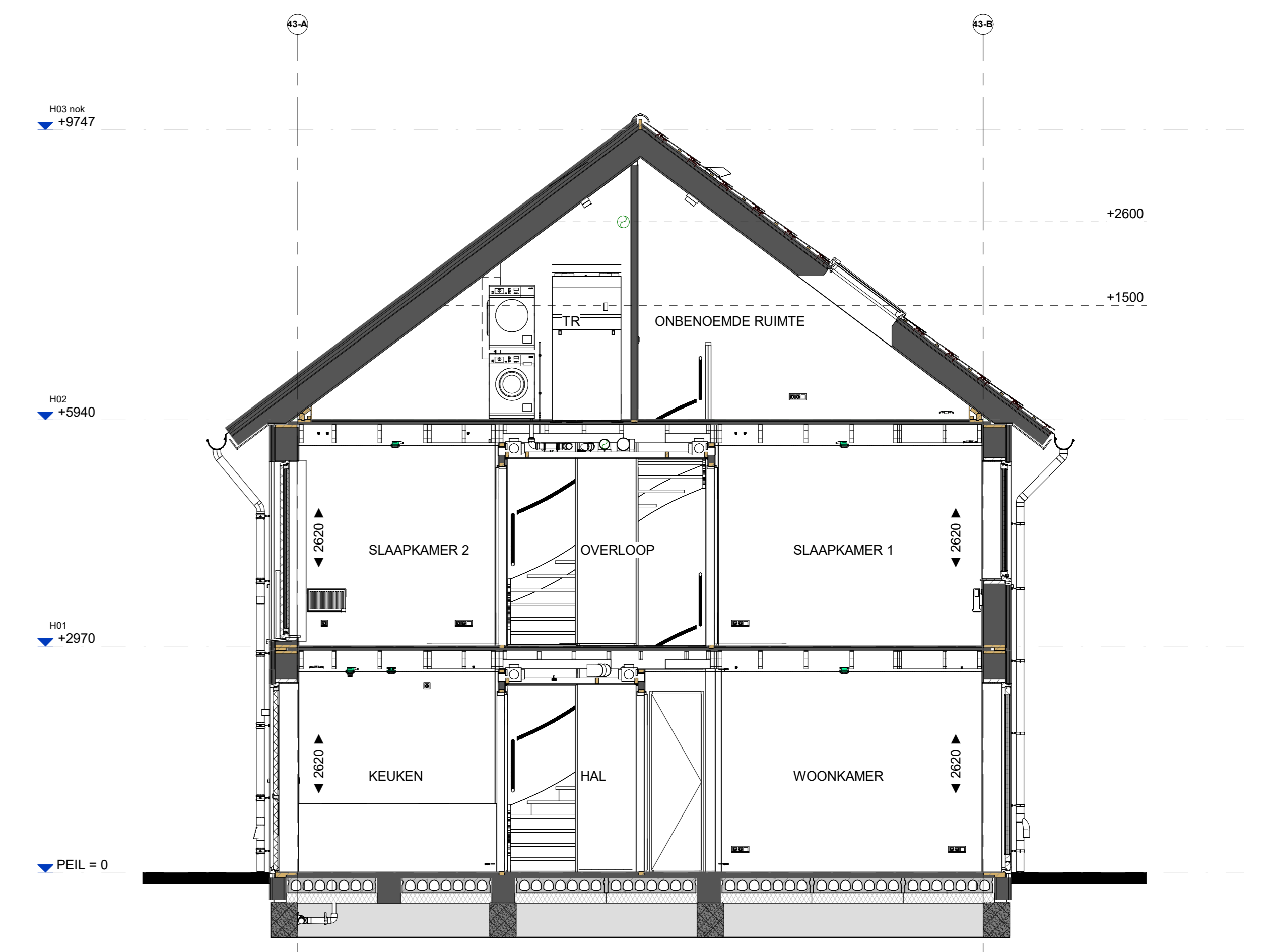
Doorsnede V01
