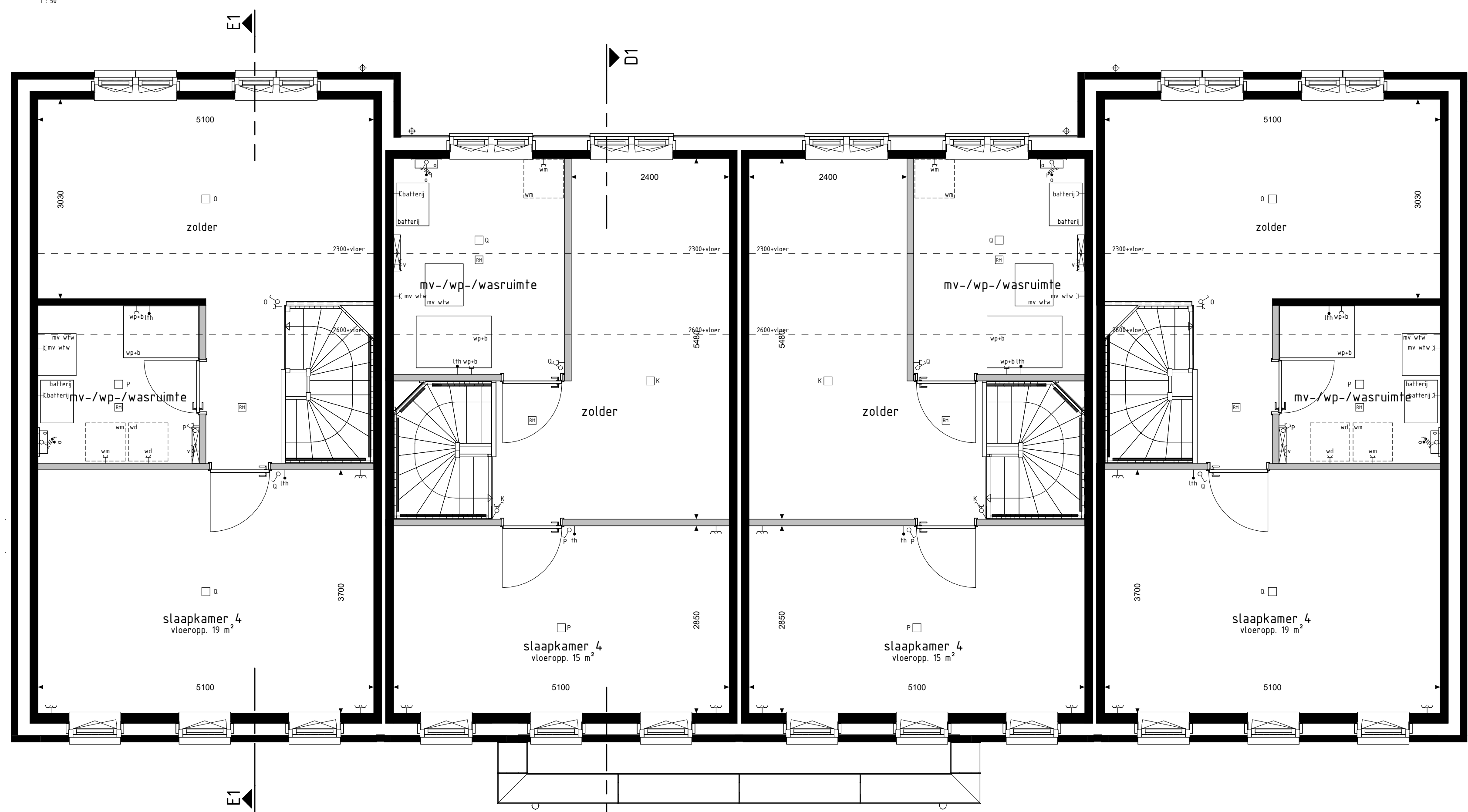
type E1 bwnr get.: 15, 19, 23 2e VERDIEPING 1:50
