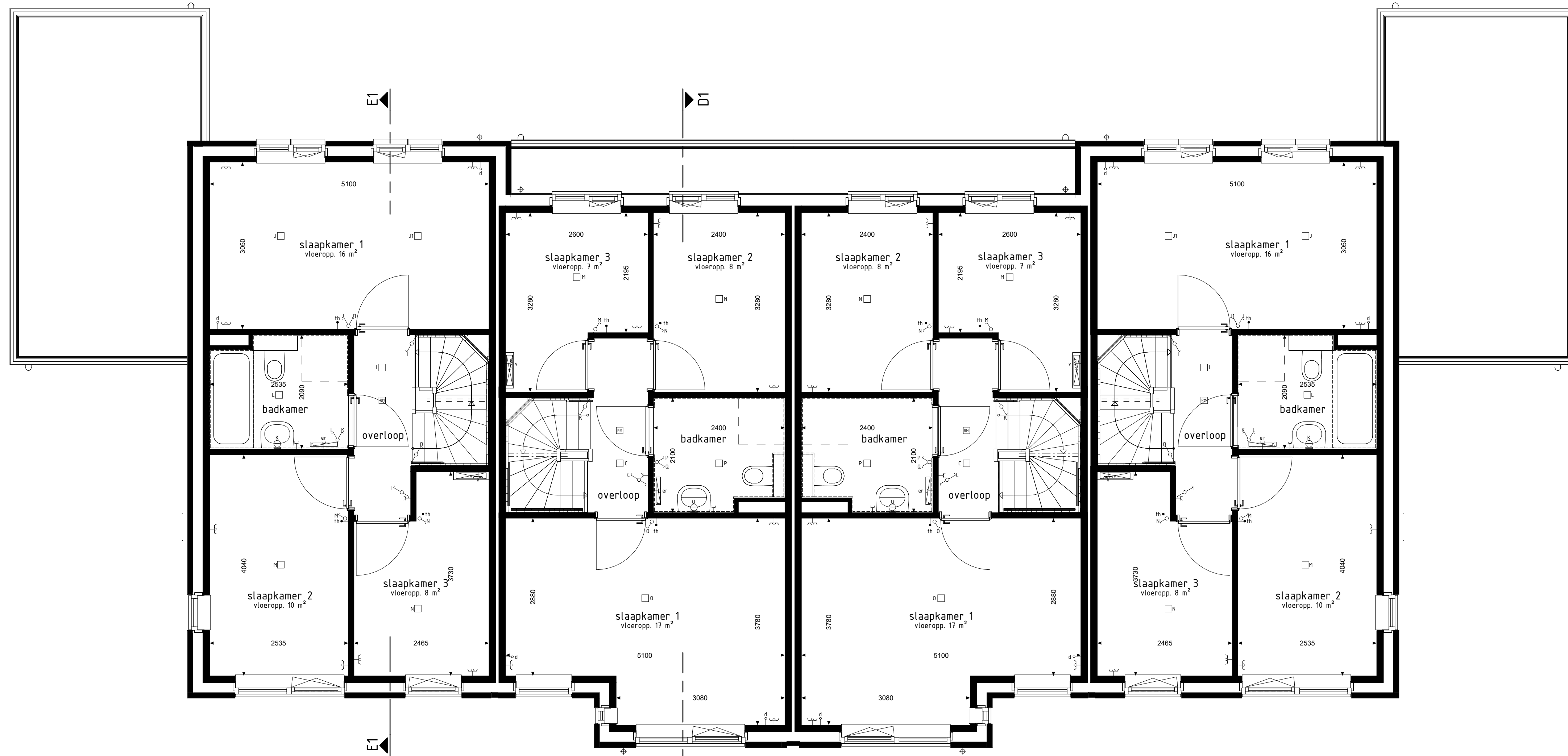
type E1 bwnr get.: 15, 19, 23 1e VERDIEPING 1:50
