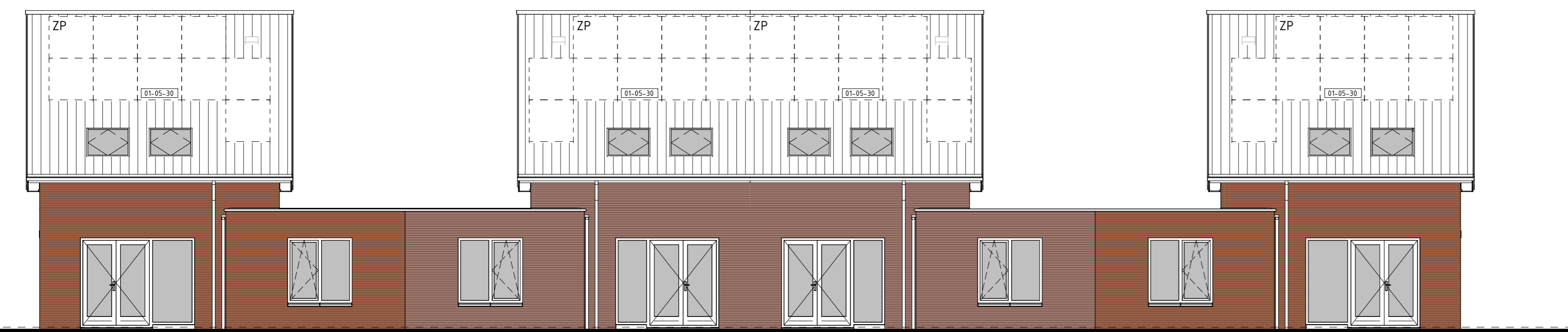
type H1 bwnr get.:14 ACHTERGEVEL 1:100
