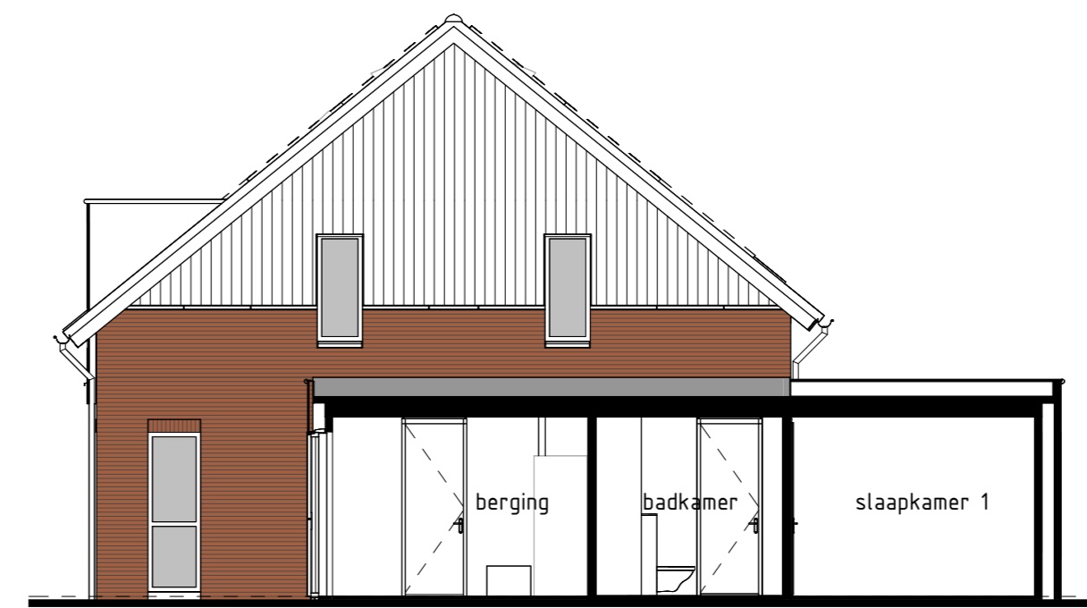
type H1, H1sp bwnr get.:14 type G2sp bwnr get.:13 RECHTERGEVEL 1:100
