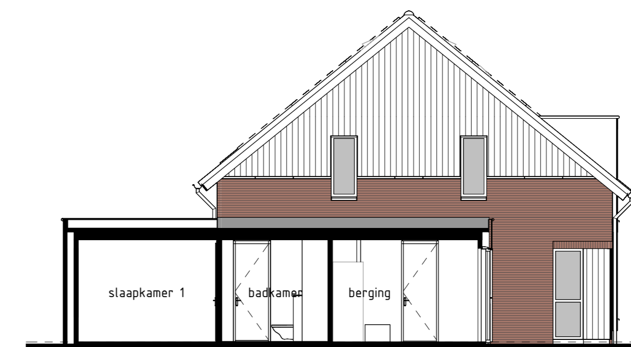
type G1 bwnr get.:12 LINKERGEVEL 1:100
