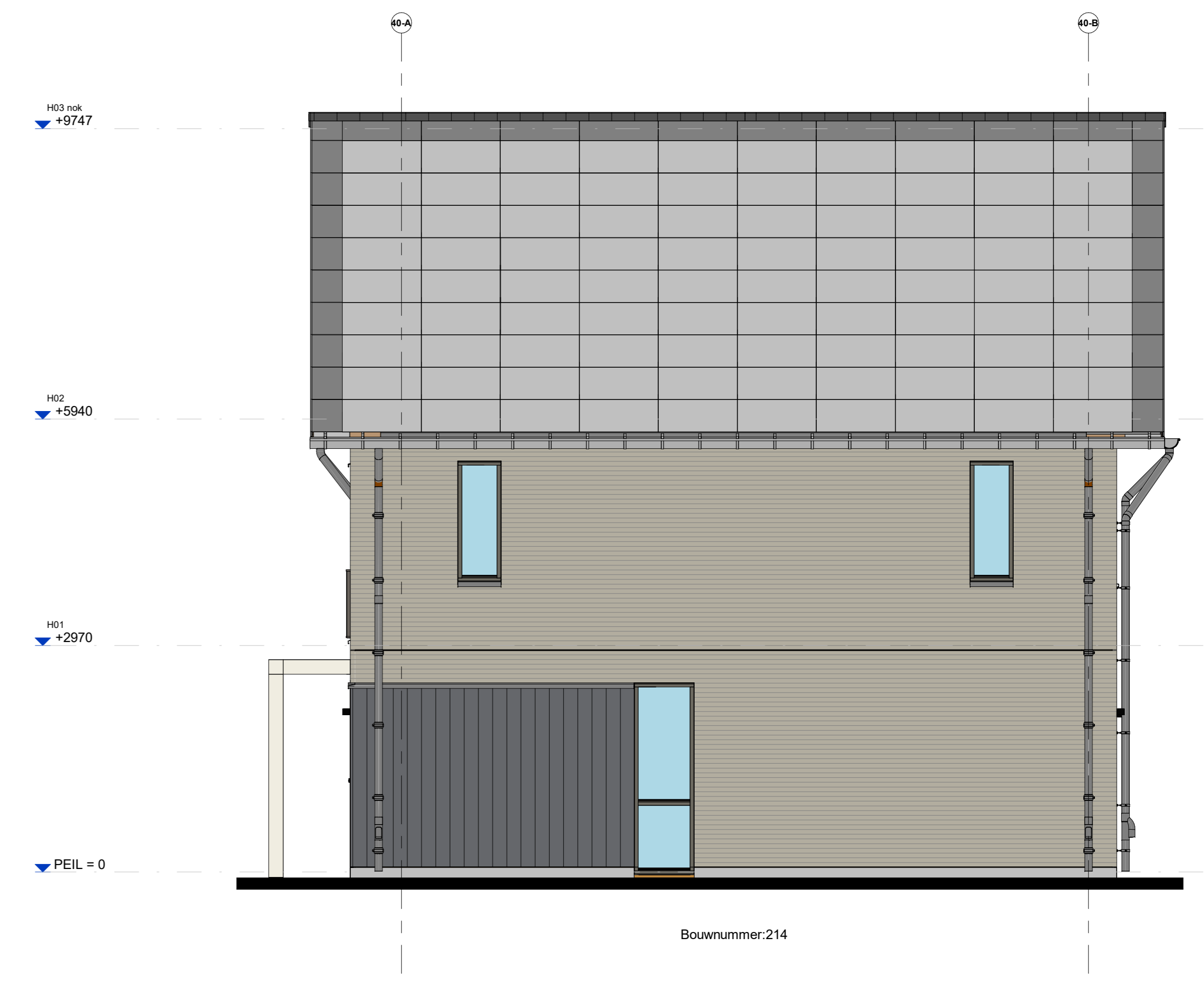
Blok 40 - Rechtergevel
