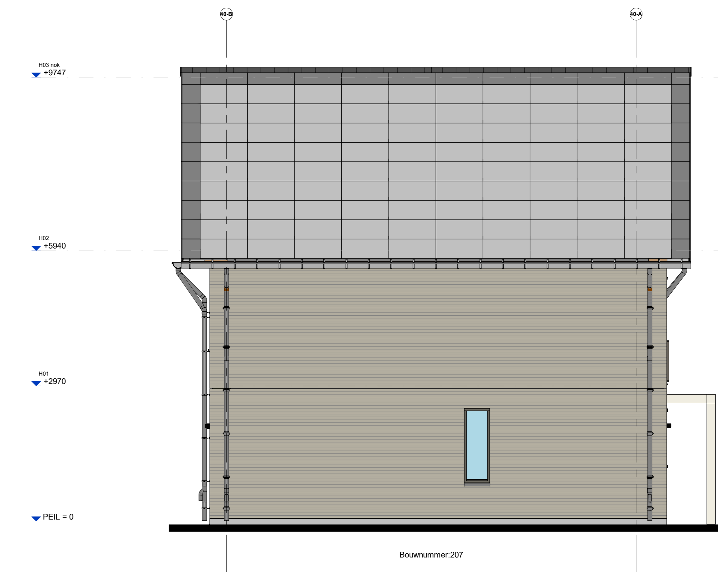
Blok 40 - Linkergevel
