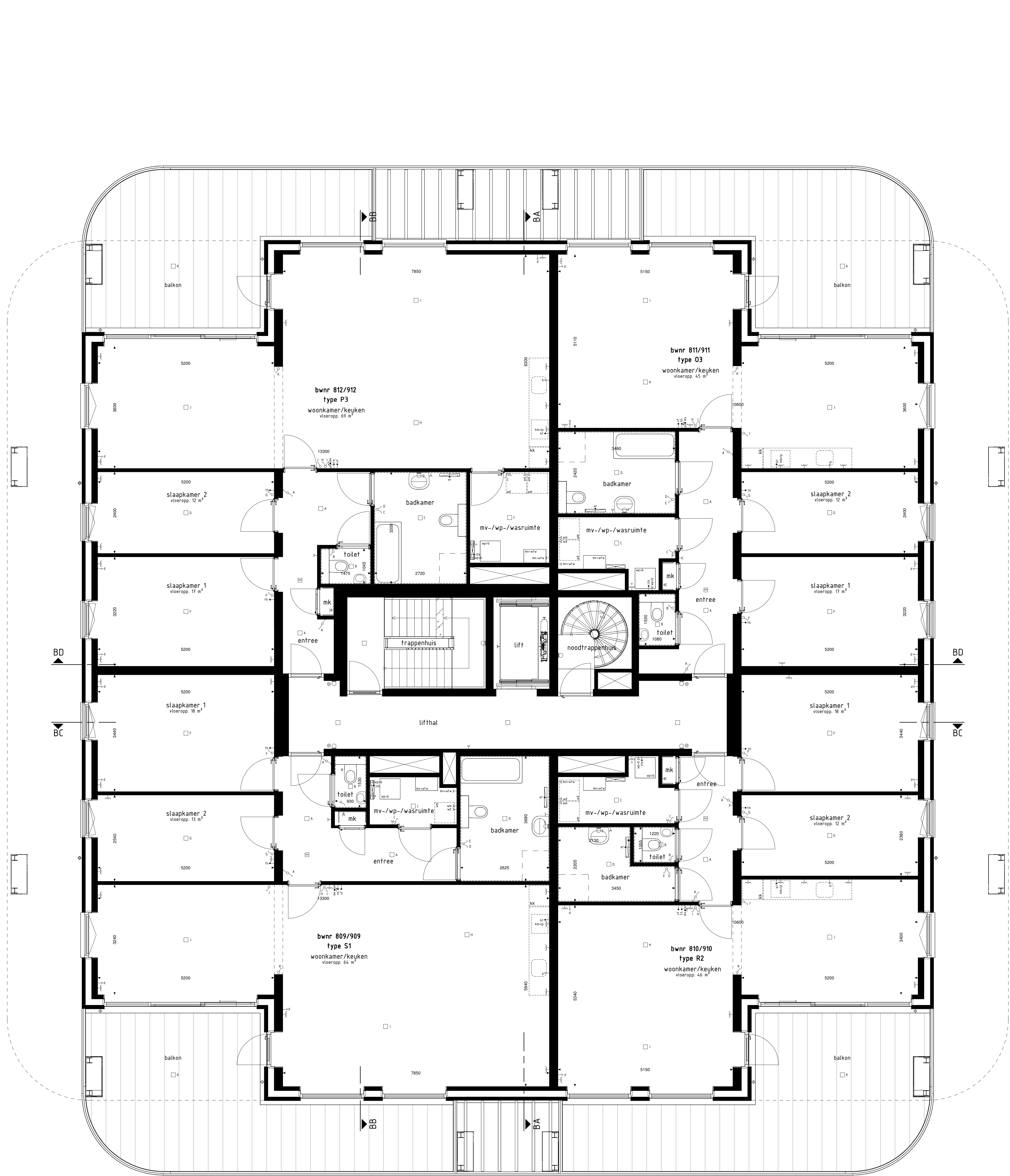
2e VERDIEPING 1:50
