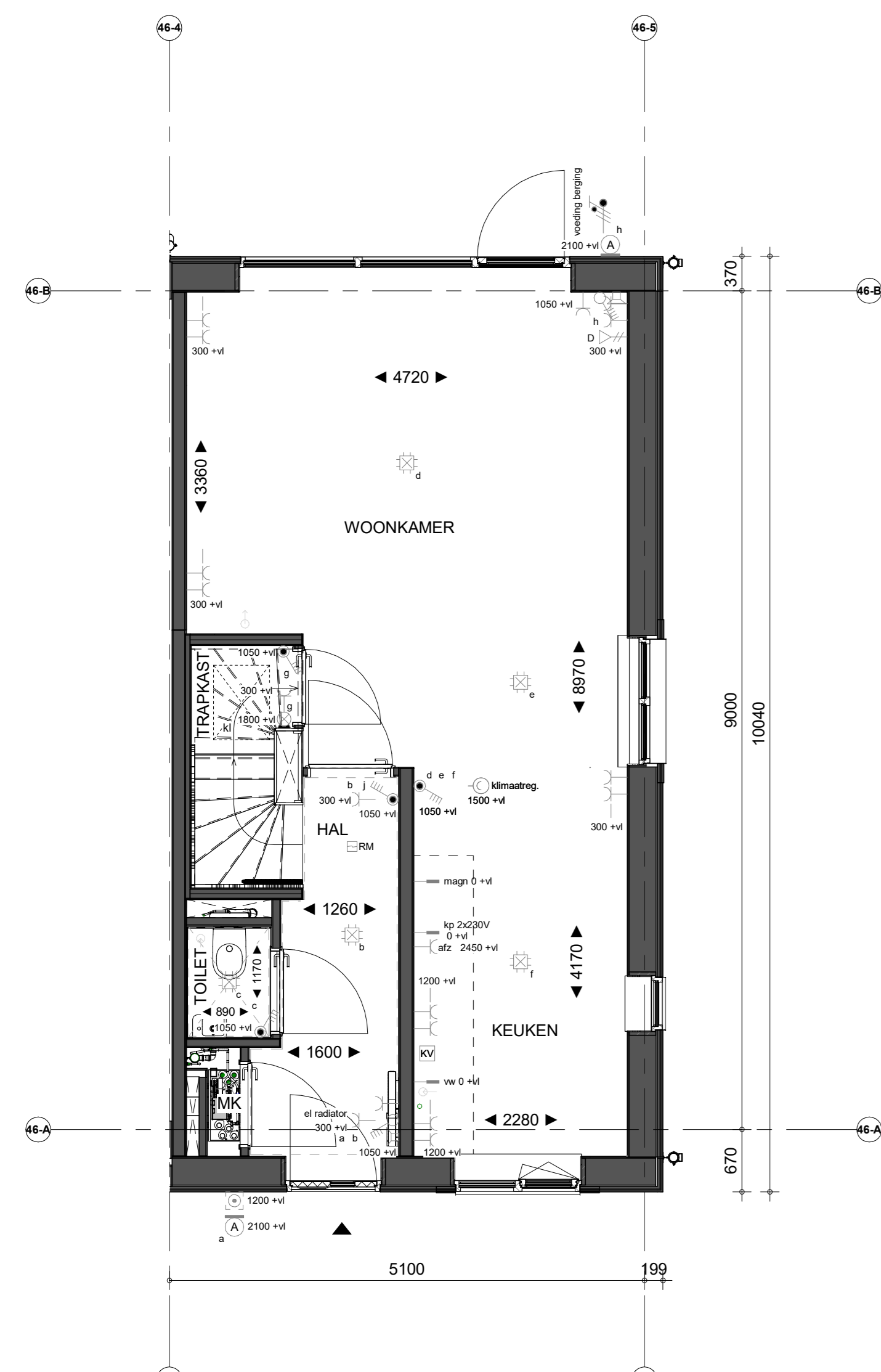
Begane grond
