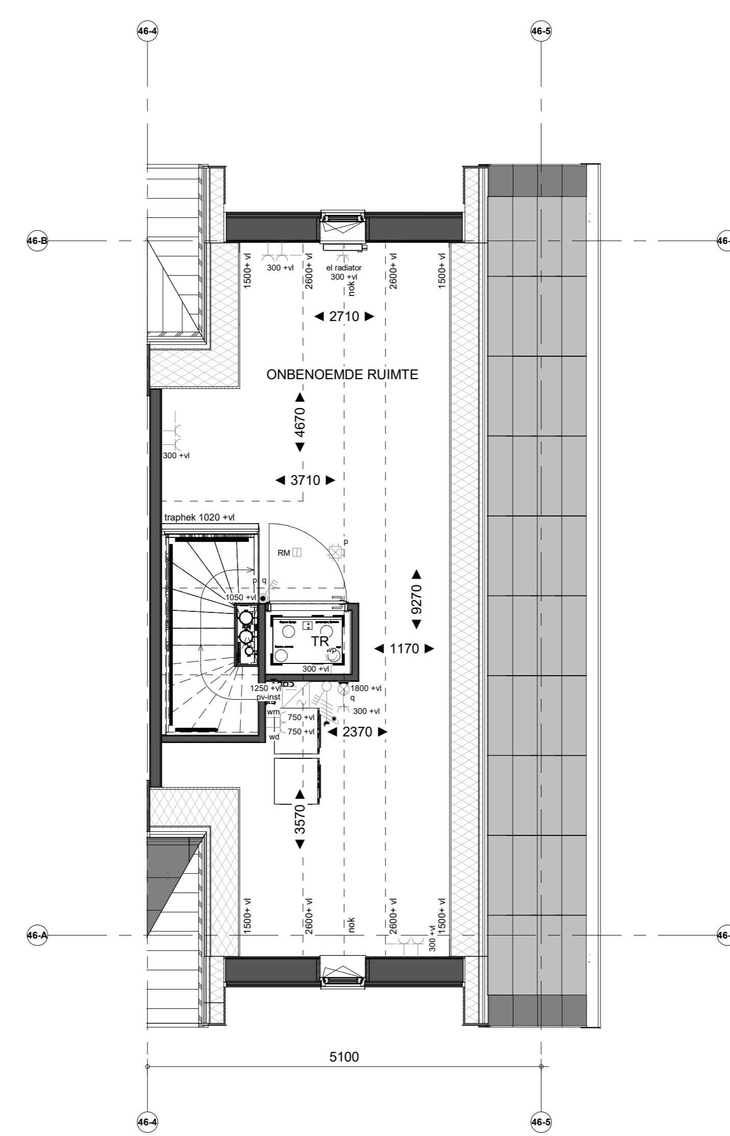
2e Verdieping
