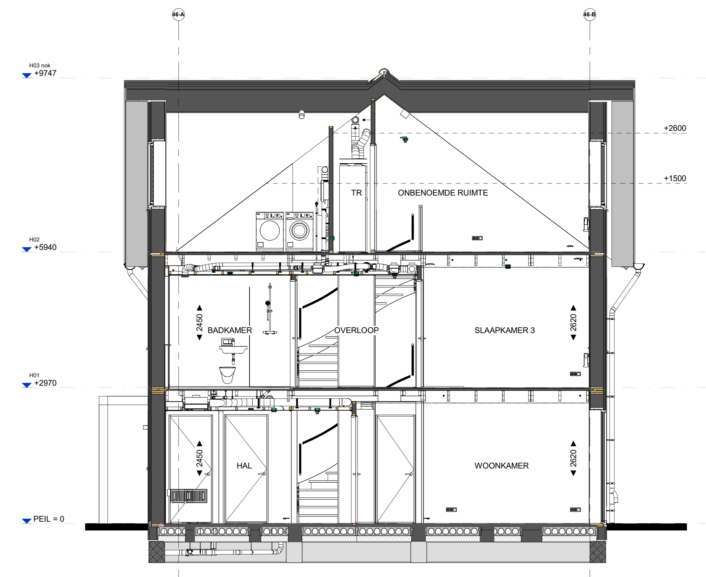
Doorsnede V01
