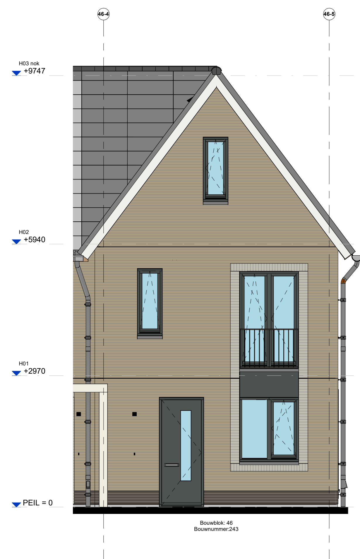
Voorgevel
