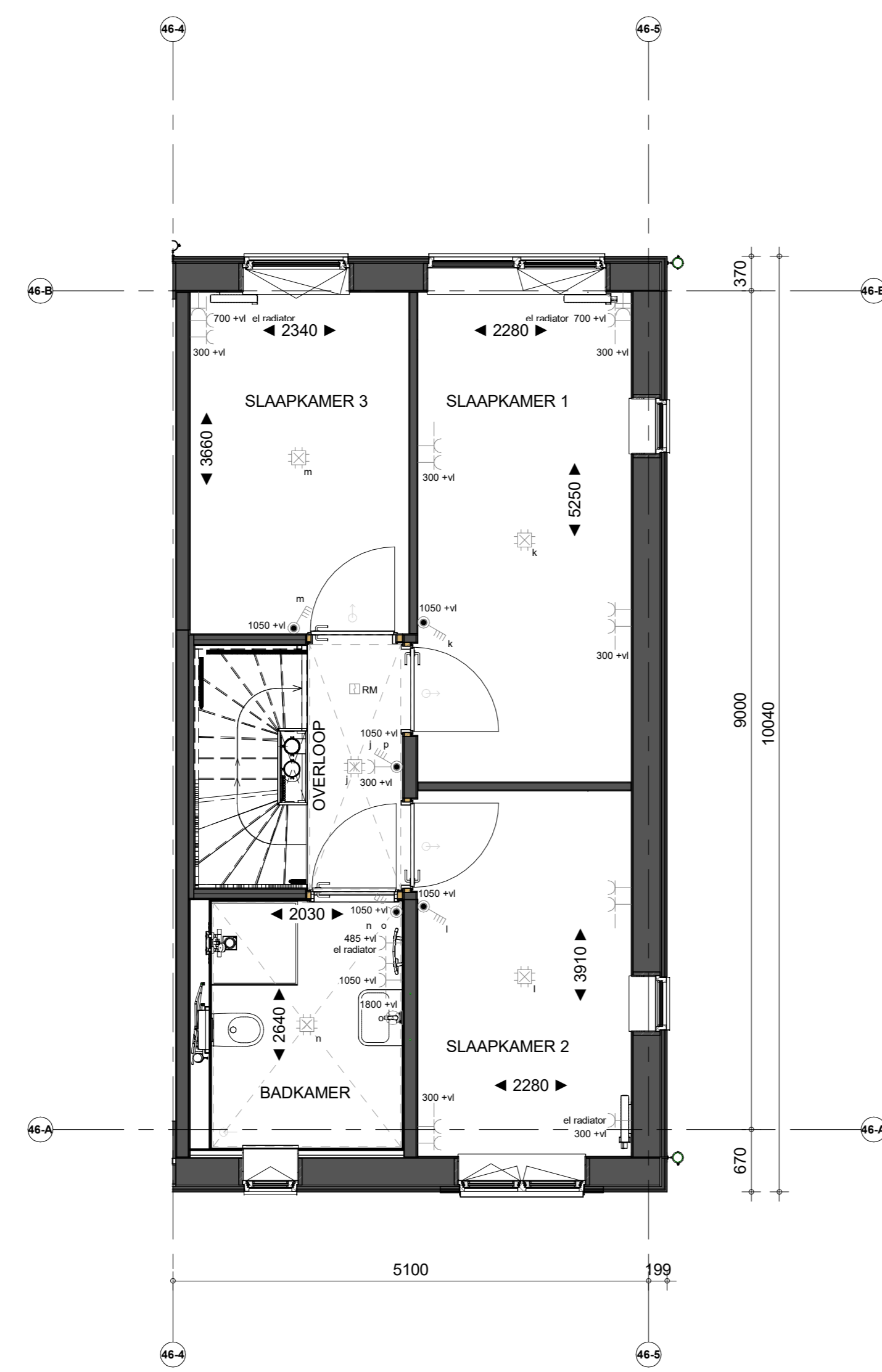
1e Verdieping
