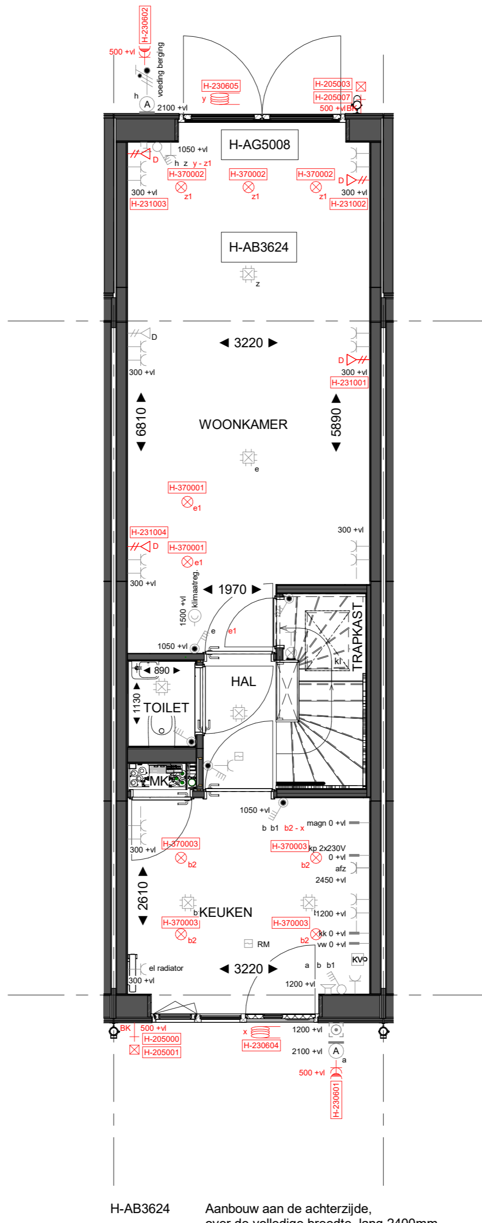
H-AB3624 Aanbouw aan de achterzijde, over de volledige breedte, lang 2400mm H-AG5008 Achtergevel voorzien van dubbele openslaande deuren
