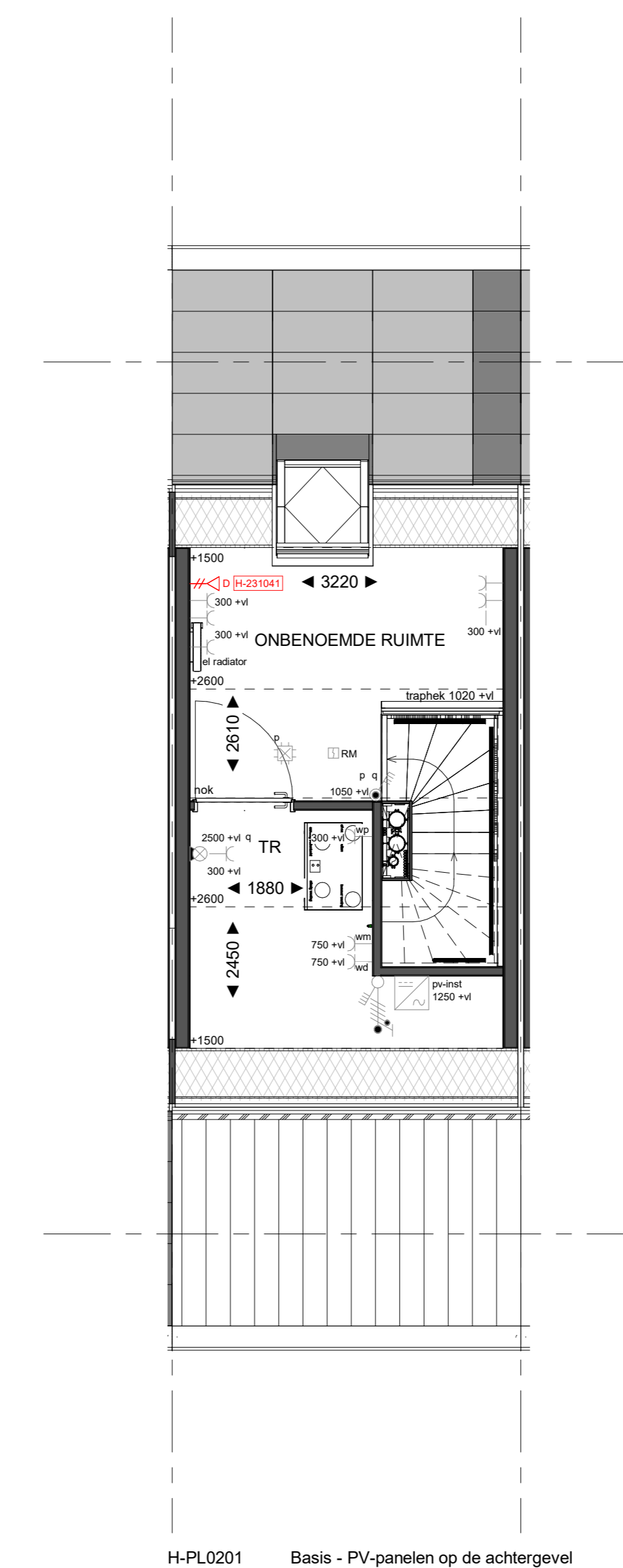
H-PL0201 Basis - PV-panelen op de achtergevel
