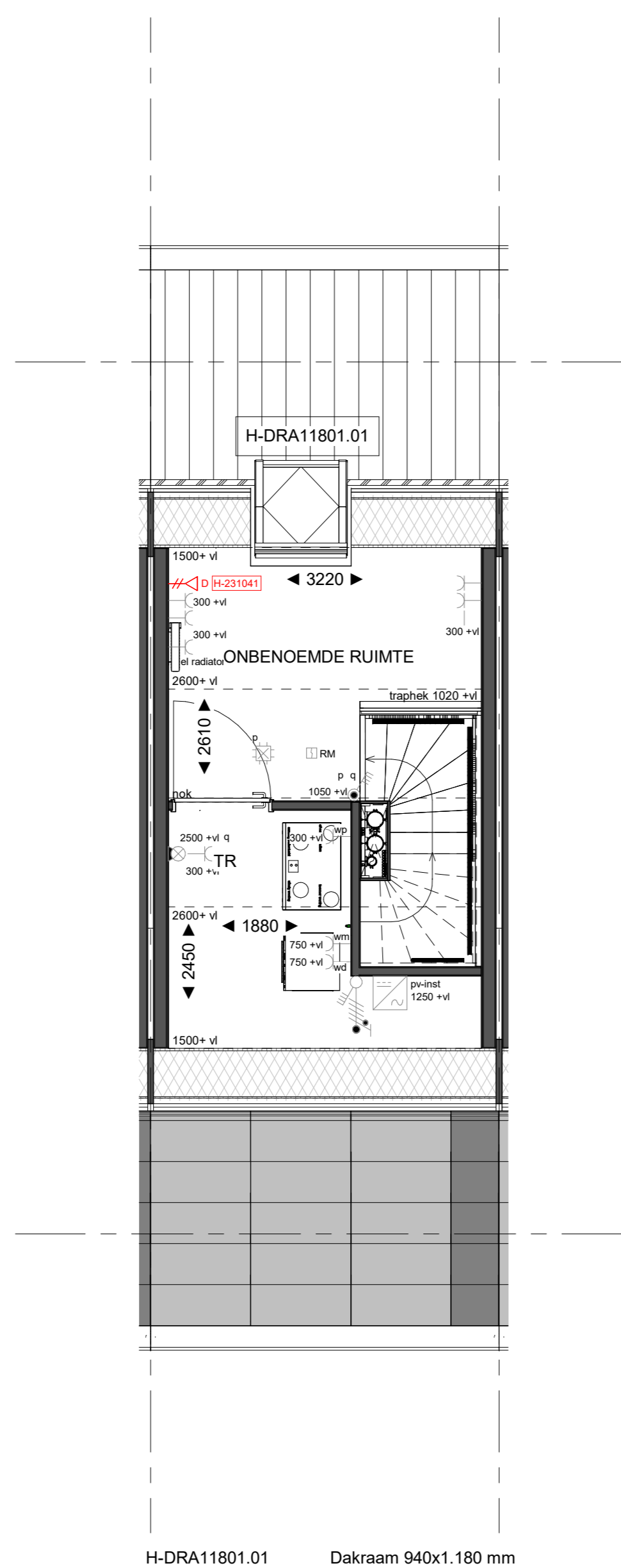
H-DRA11801.01 Dakraam 940x1.180 mm in de achtergevel l.p.v. de onbenoemde ruimte (boven slaapkamer 1) i.p.v. klein dakraam
