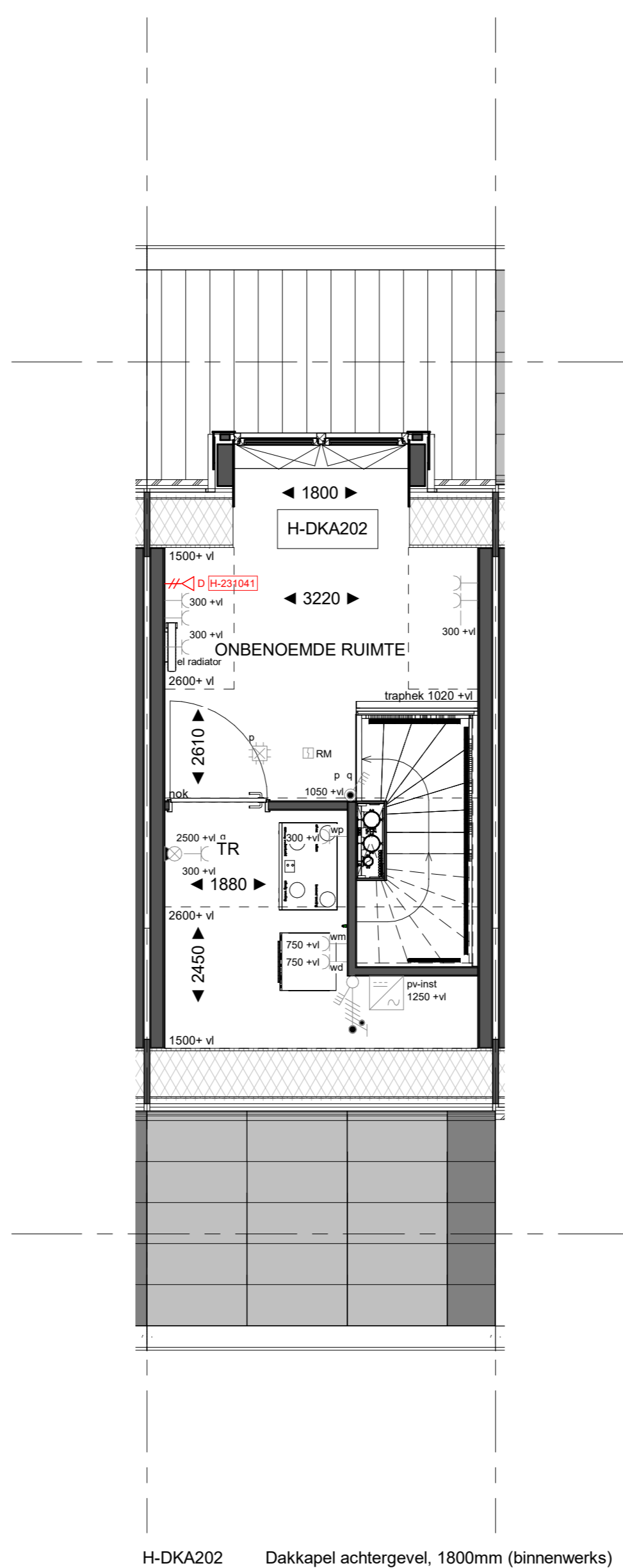
H-DKA202 Dakkapel achtergevel, 1800mm (binnenwerks) met overstek. Optie mogelijk afhankelijk van positie PV-panelen
